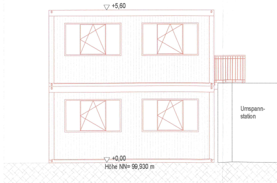
Bürocontainer Position 1, Ansicht Süd-West, M. 1:100
