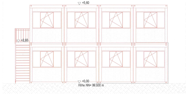
Bürocontainer Position 1, Ansicht Nord-West, M. 1:100
