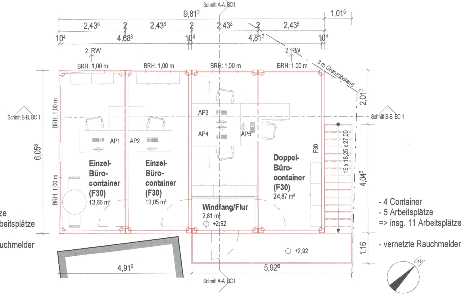
Bürocontainer Position 1, Grundriss Obergeschoss, M. 1:100
