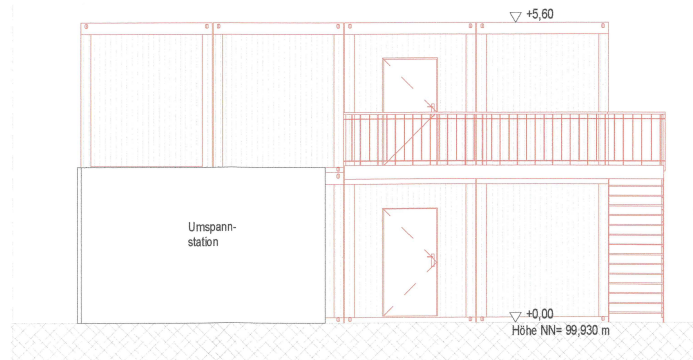
Bürocontainer Position 1, Ansicht Süd-Ost, M. 1:100
