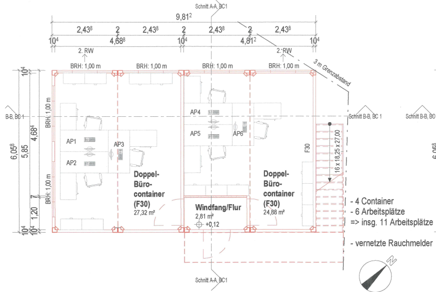
Bürocontainer Position 1, Grundriss Erdgeschoss, M. 1:100
