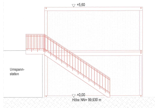
Bürocontainer Position 1, Ansicht Nord-Ost, M. 1:100
