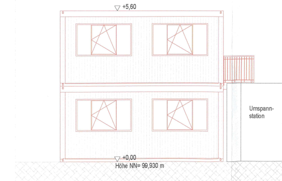
Bürocontainer Position 1, Ansicht Süd-West, M. 1:100
