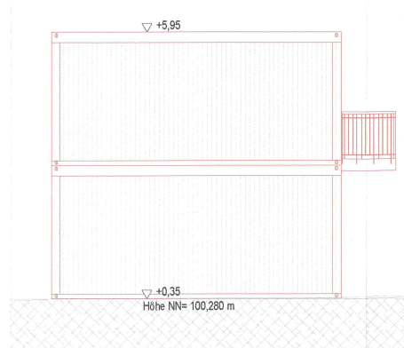
Bürocontainer Position 2, Ansicht Süd-West, M. 1:100
