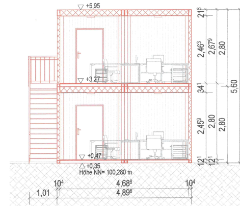
Bürocontainer Position 2, Schnitt B-B, M. 1:100
