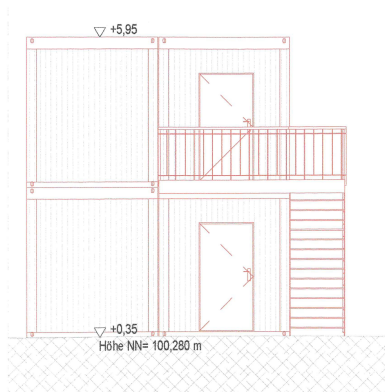
Bürocontainer Position 2, Ansicht Süd-Ost, M. 1:100
