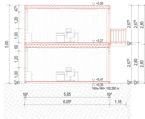
Bürocontainer Position 2, Schnitt A-A, M. 1:100
