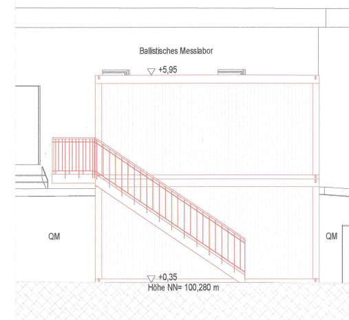
Bürocontainer Position 2, Ansicht Nord-Ost, M. 1:100
