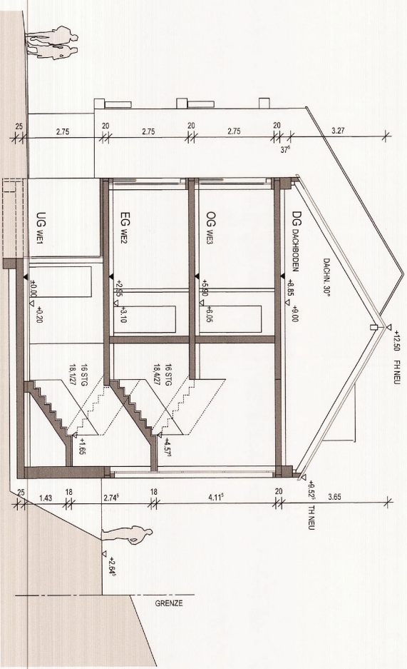
SCHNITT A-A
