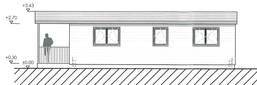
Ansicht Süd
