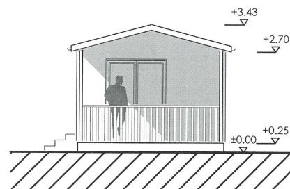
Ansicht West
