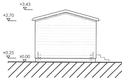
Ansicht Ost
