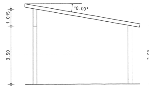
Schnitt B-B
