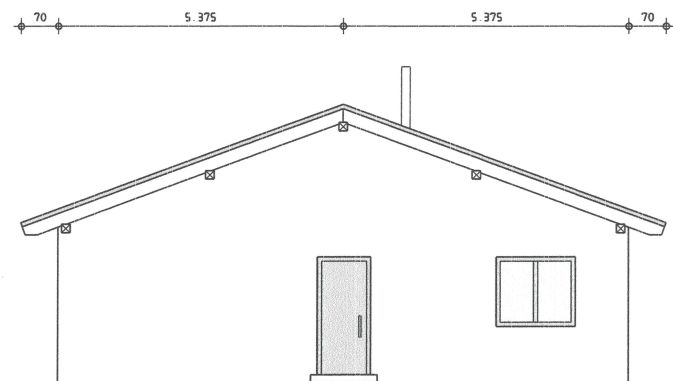
Ansicht Nord-Ost
