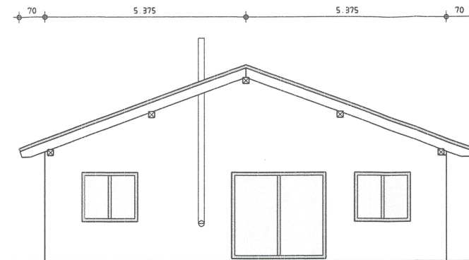
Ansicht Süd-West
