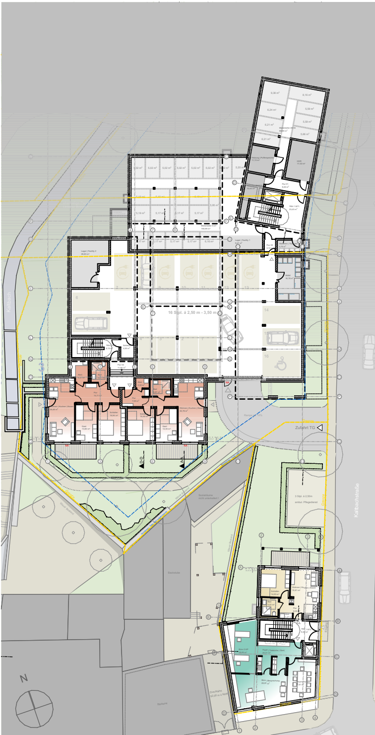
Grundriss Erdgeschoss
