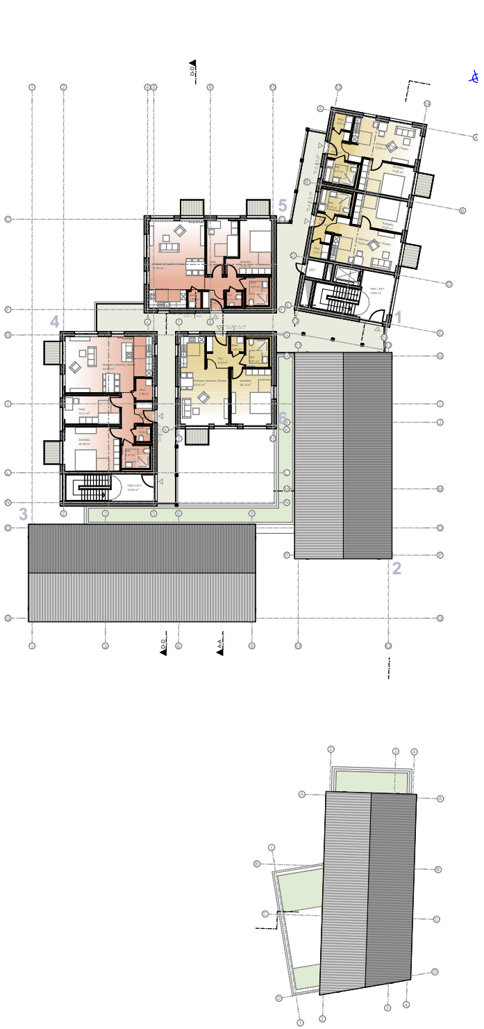
Grundriss 3.Obergeschoss
