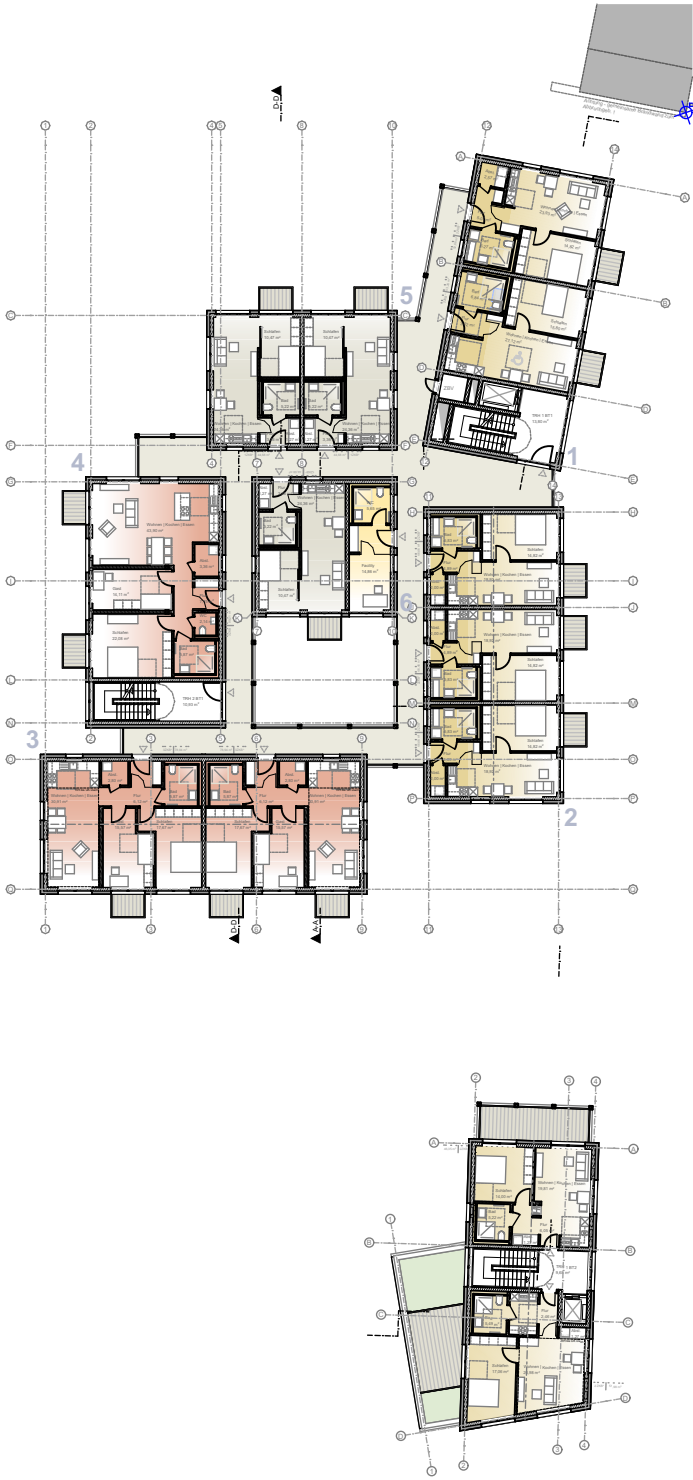
Grundriss 2.Obergeschoss
