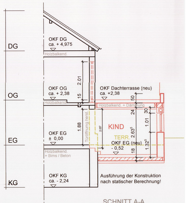
SCHNITT A-A
