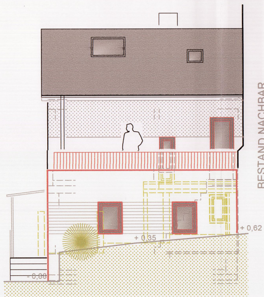
ANSICHT VON WESTEN
