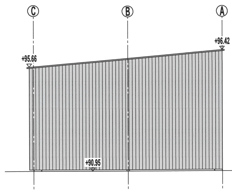
Nord - West - Ansicht
