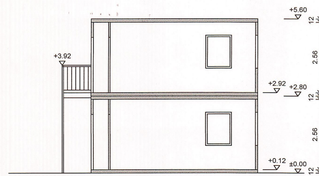
SCHNITT
