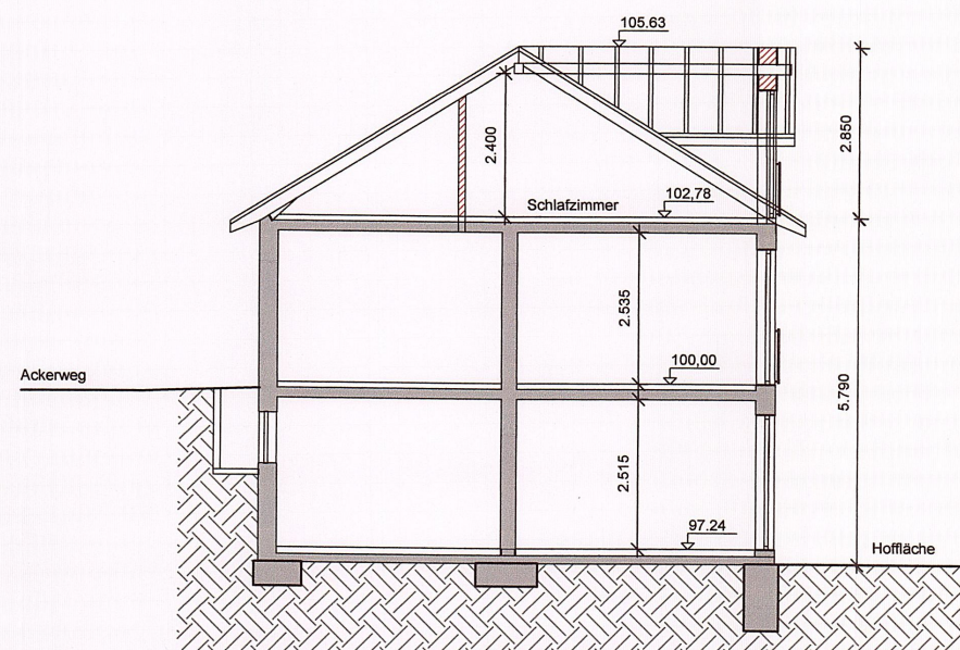
Querschnitt durch Wohnhaus mit neuem Zimmer im DG
