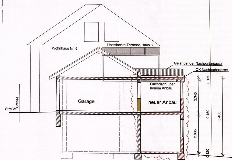
Querschnitt durch Garage mit neuem Anbau
