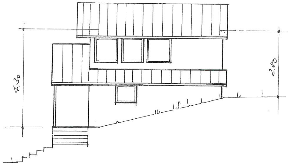
SÜD-WEST ANSICHT
