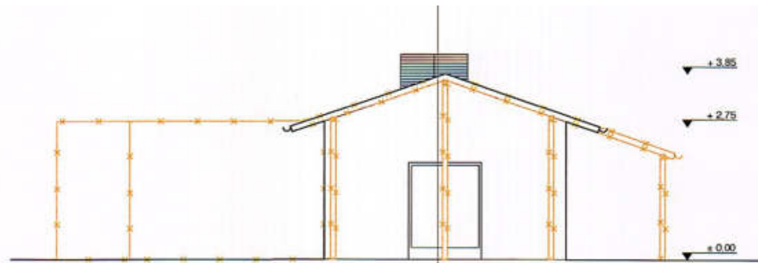
Ansicht Ost
