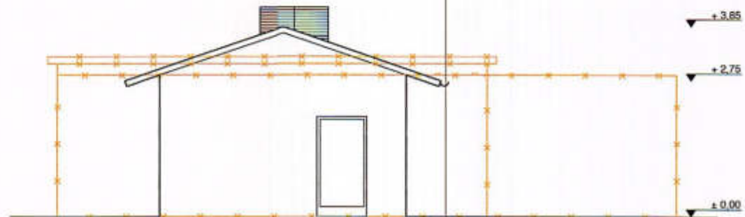
Ansicht West
