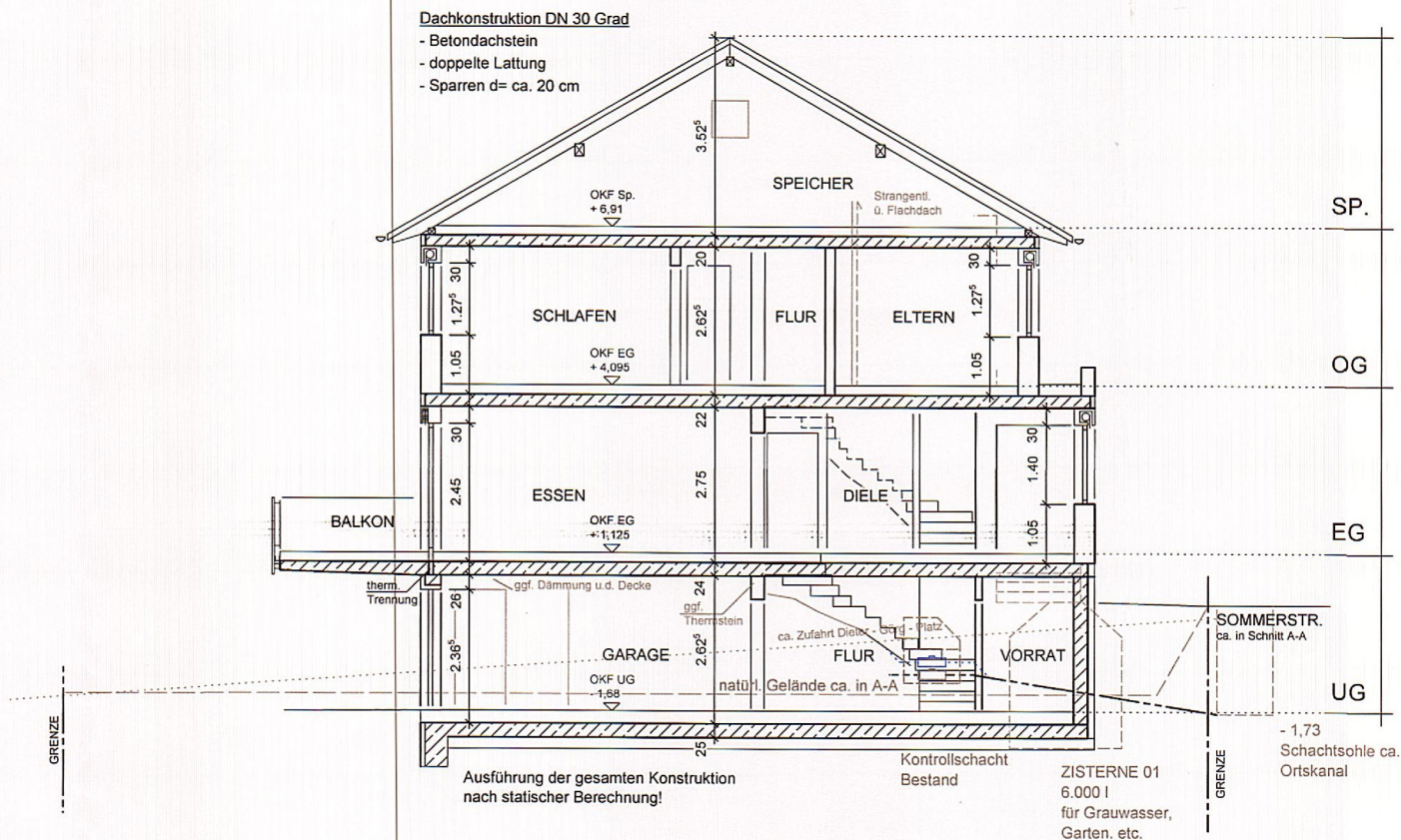
SCHNITT A - A
