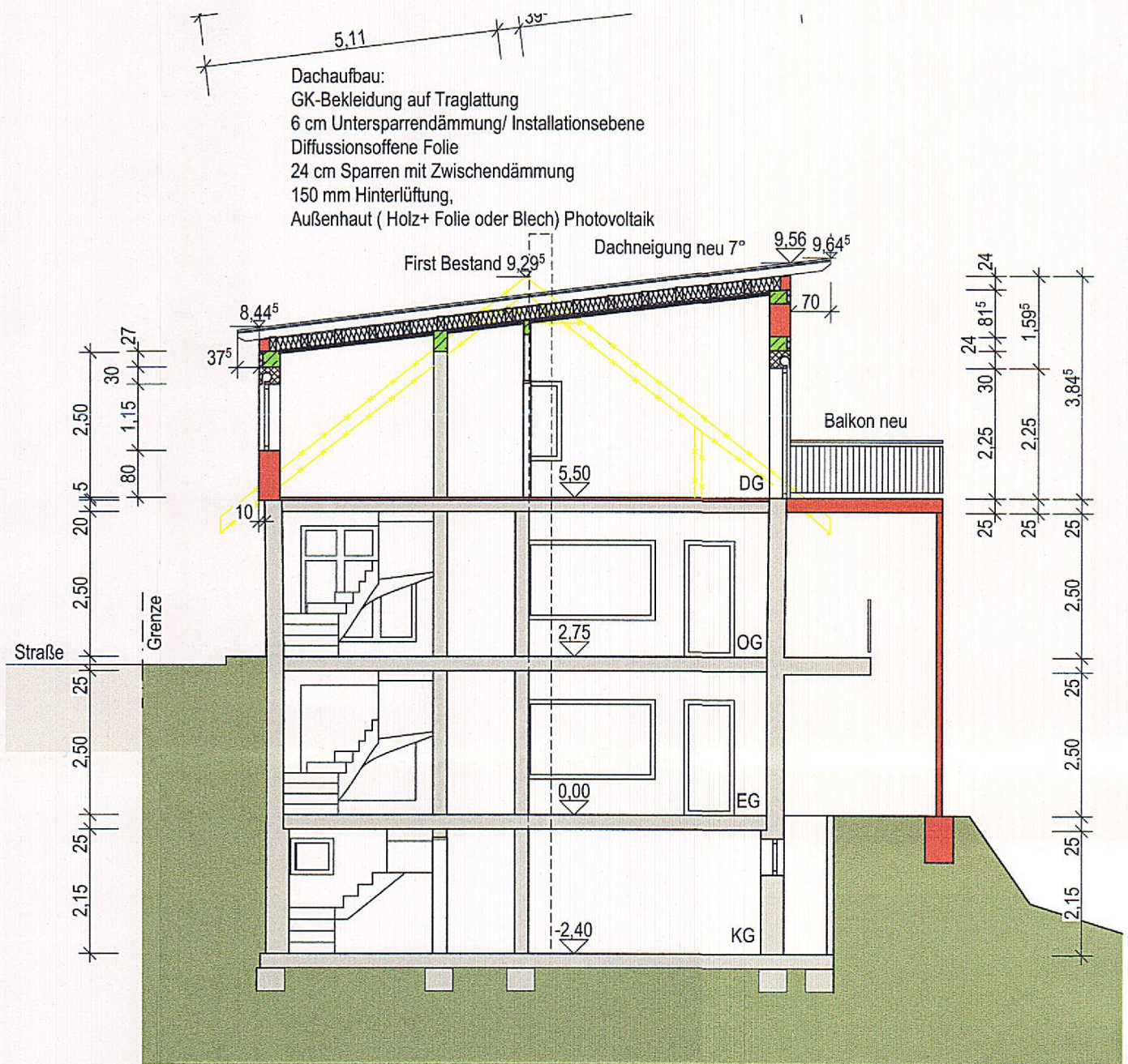
Schnitt A-A
