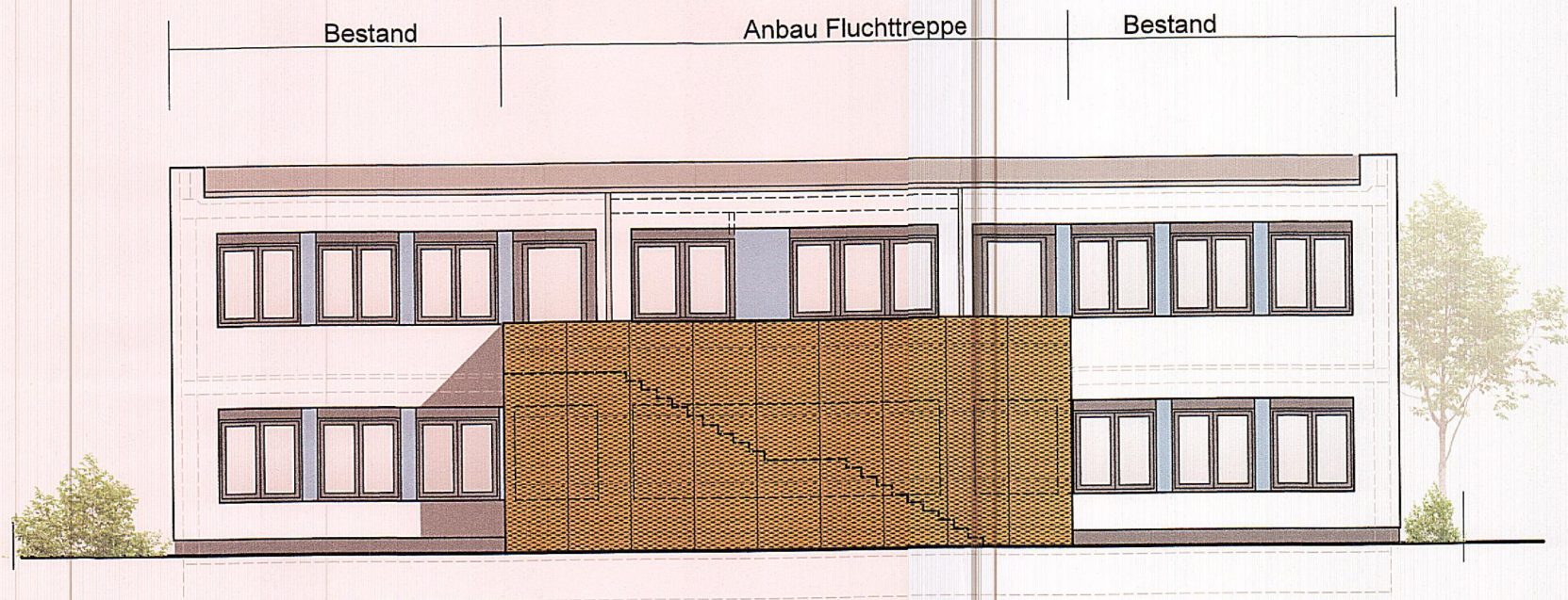
Ansicht Nord-West
