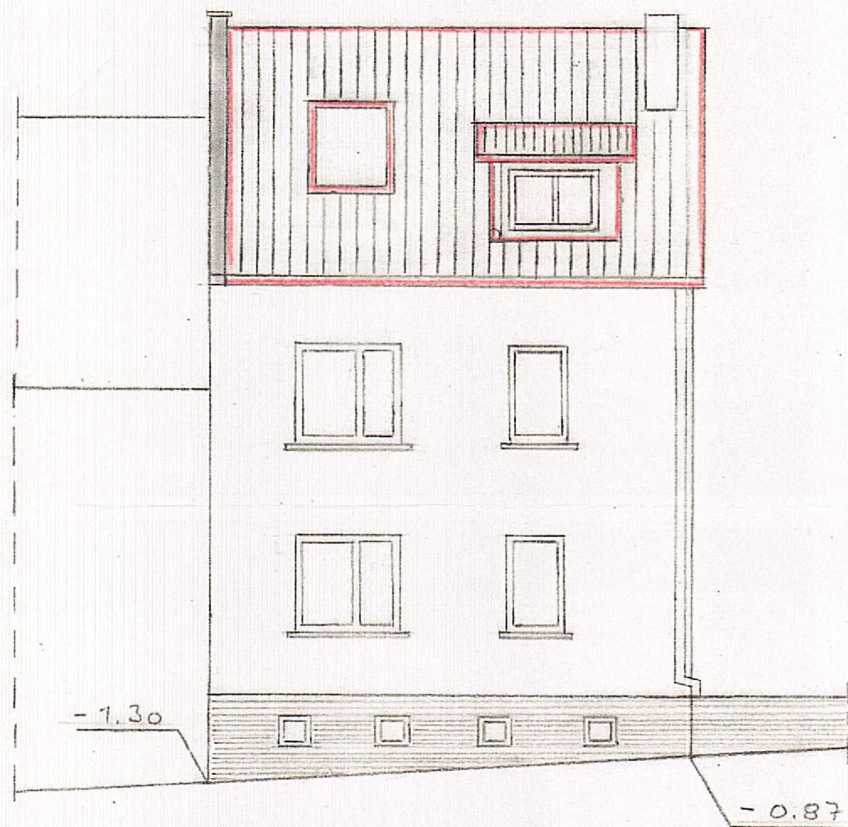
Nord-Ost Ansicht
