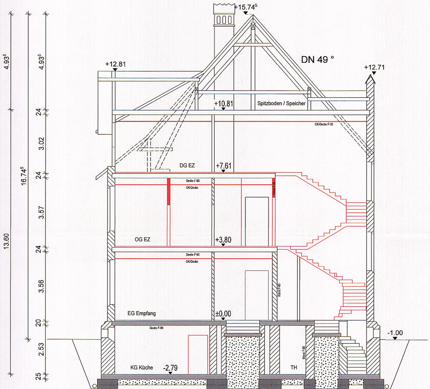
SCHNITT A-A
