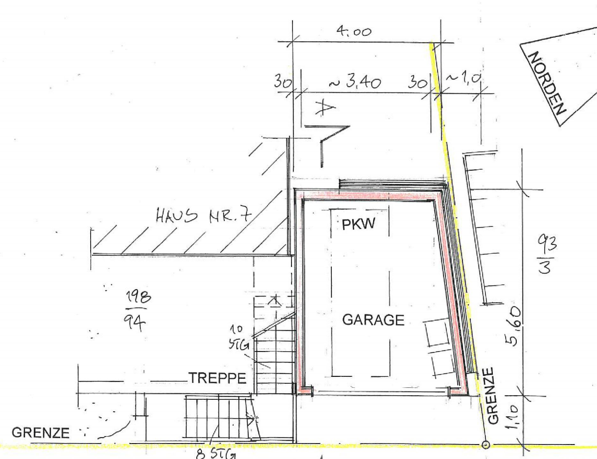
GRUNDRISS
