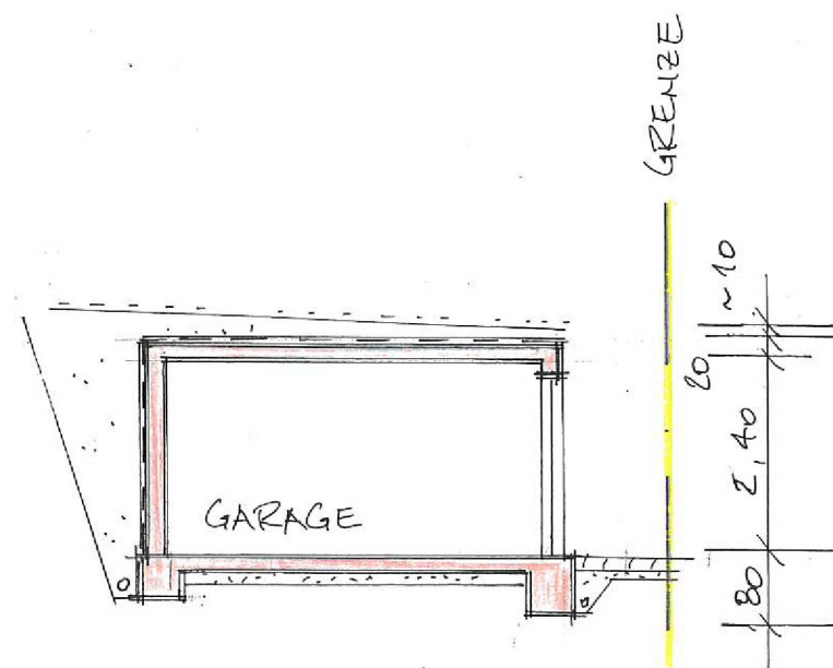
SCHNITT A-A
