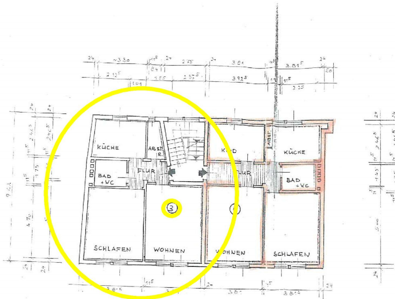
2. OBERGESCHOSS. M. 1:100
