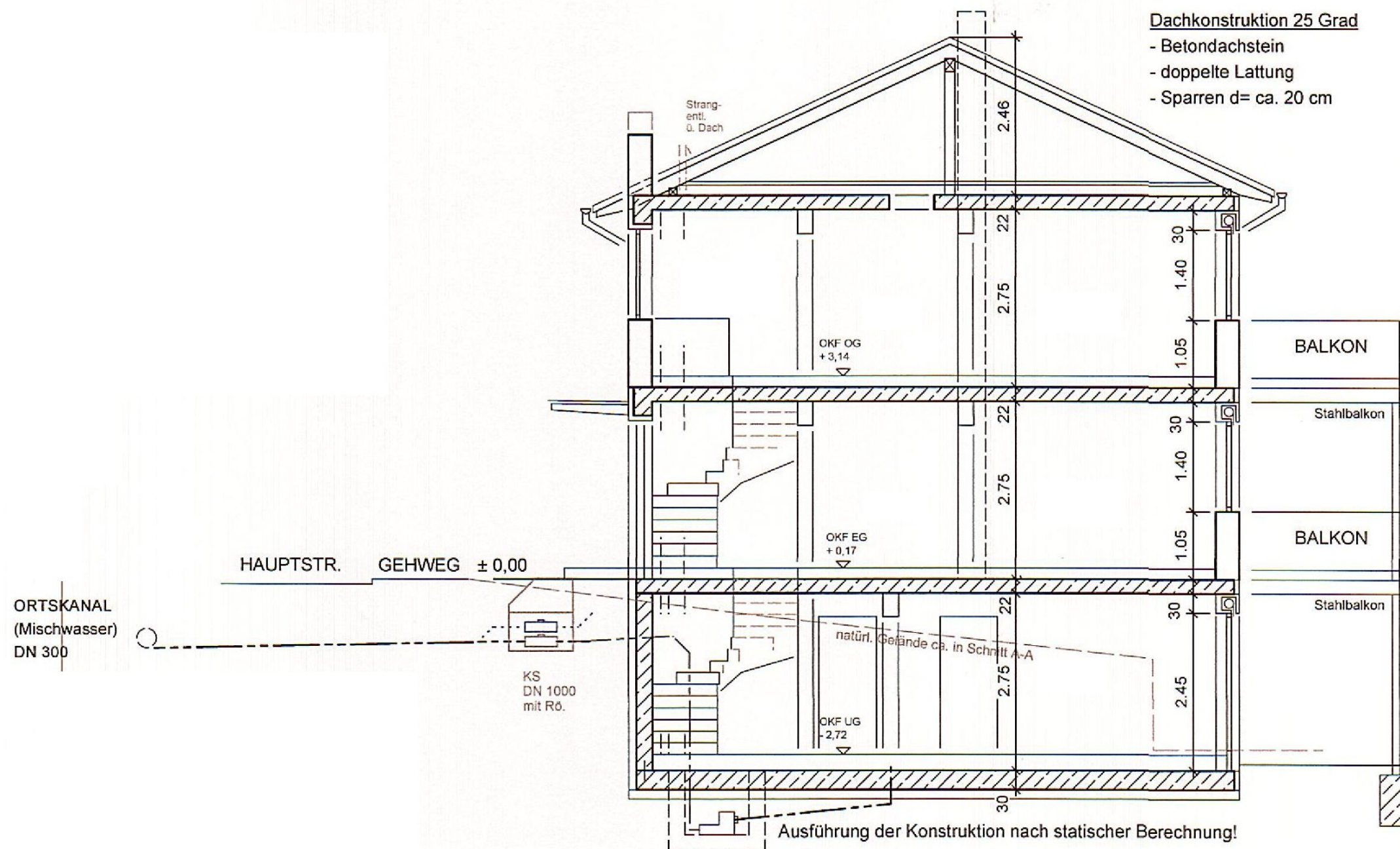
SCHNITT A - A
