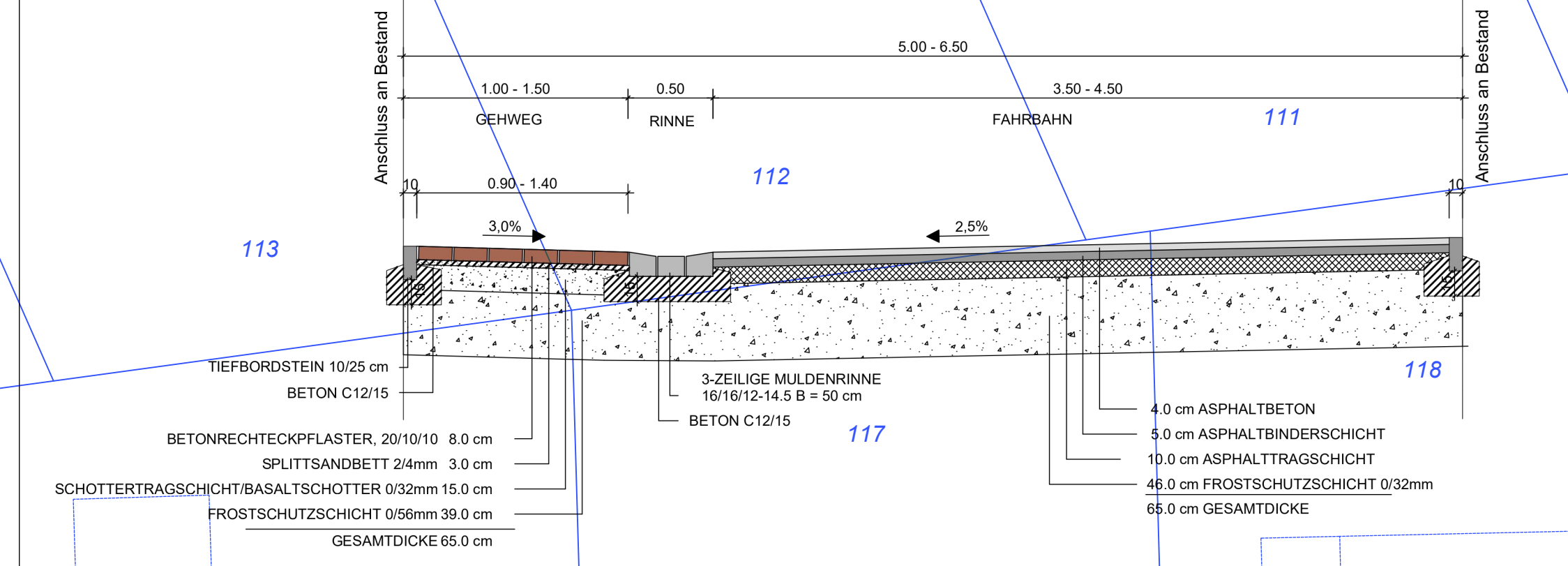
Regelquerschnitt M 1 : 25
