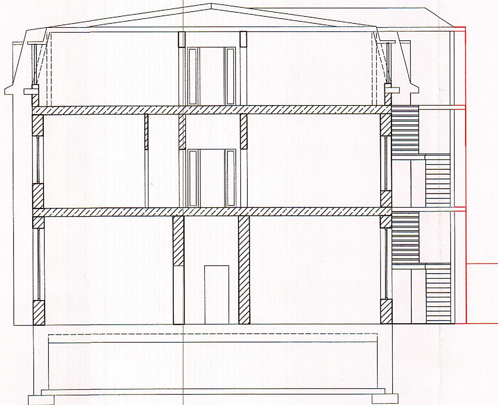
Schnitt A-A
