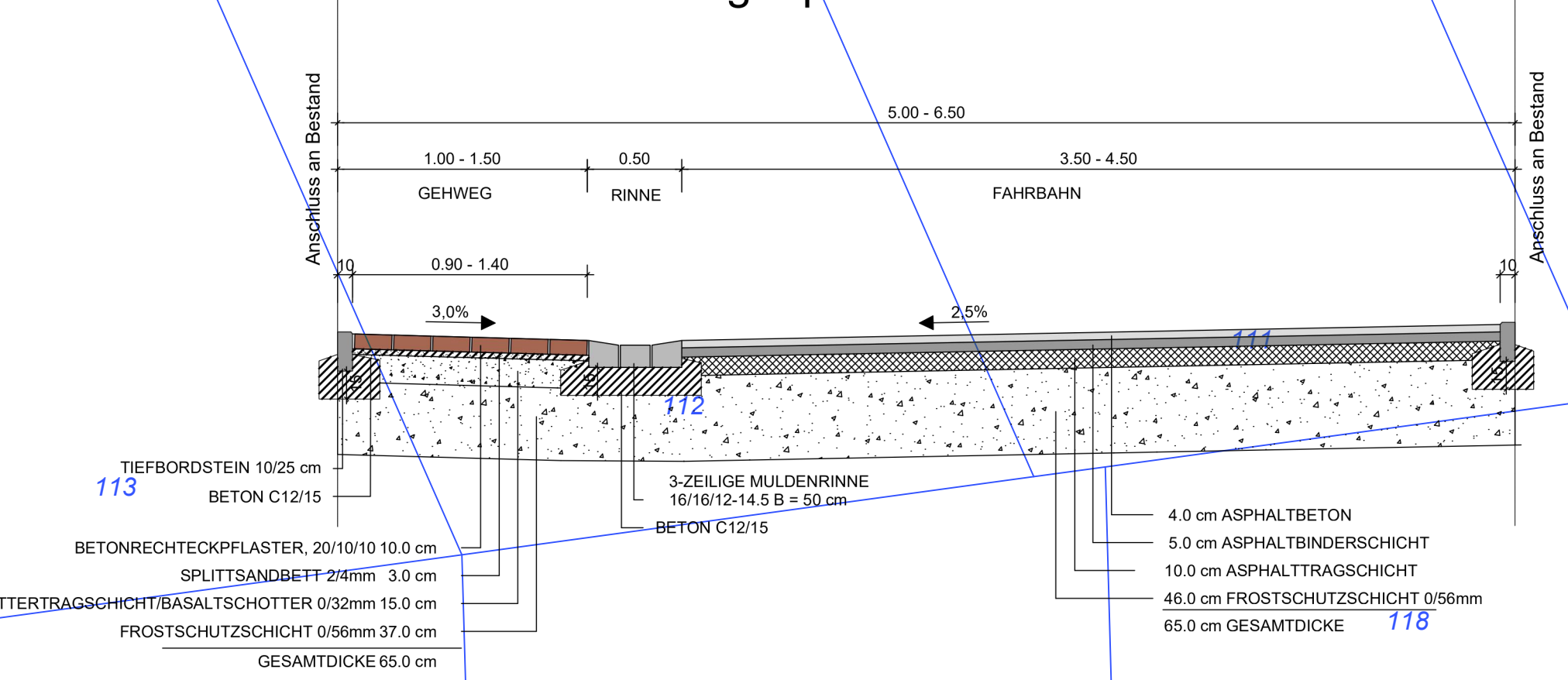
Regelquerschnitt M 1 : 25
