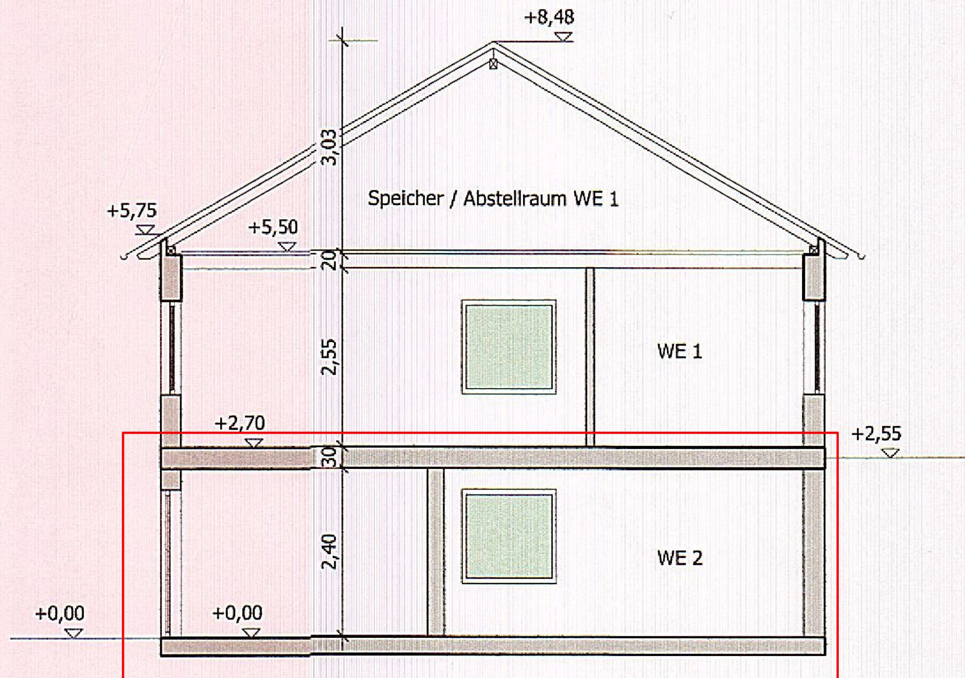
Querschnitt Bestand
