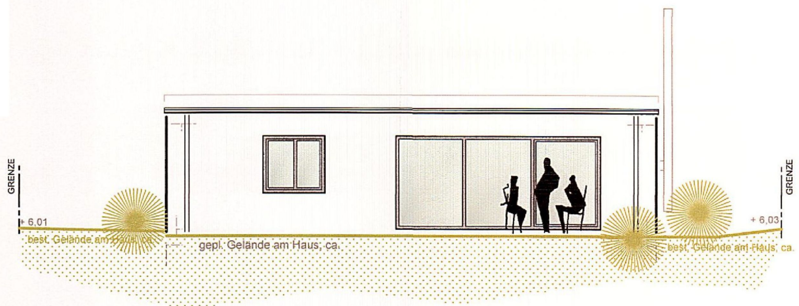
ANSICHT VON NORDEN
