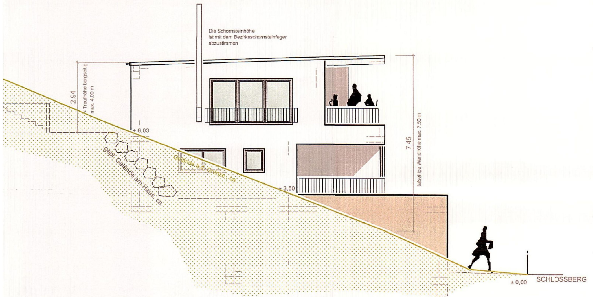
ANSICHT VON WESTEN
