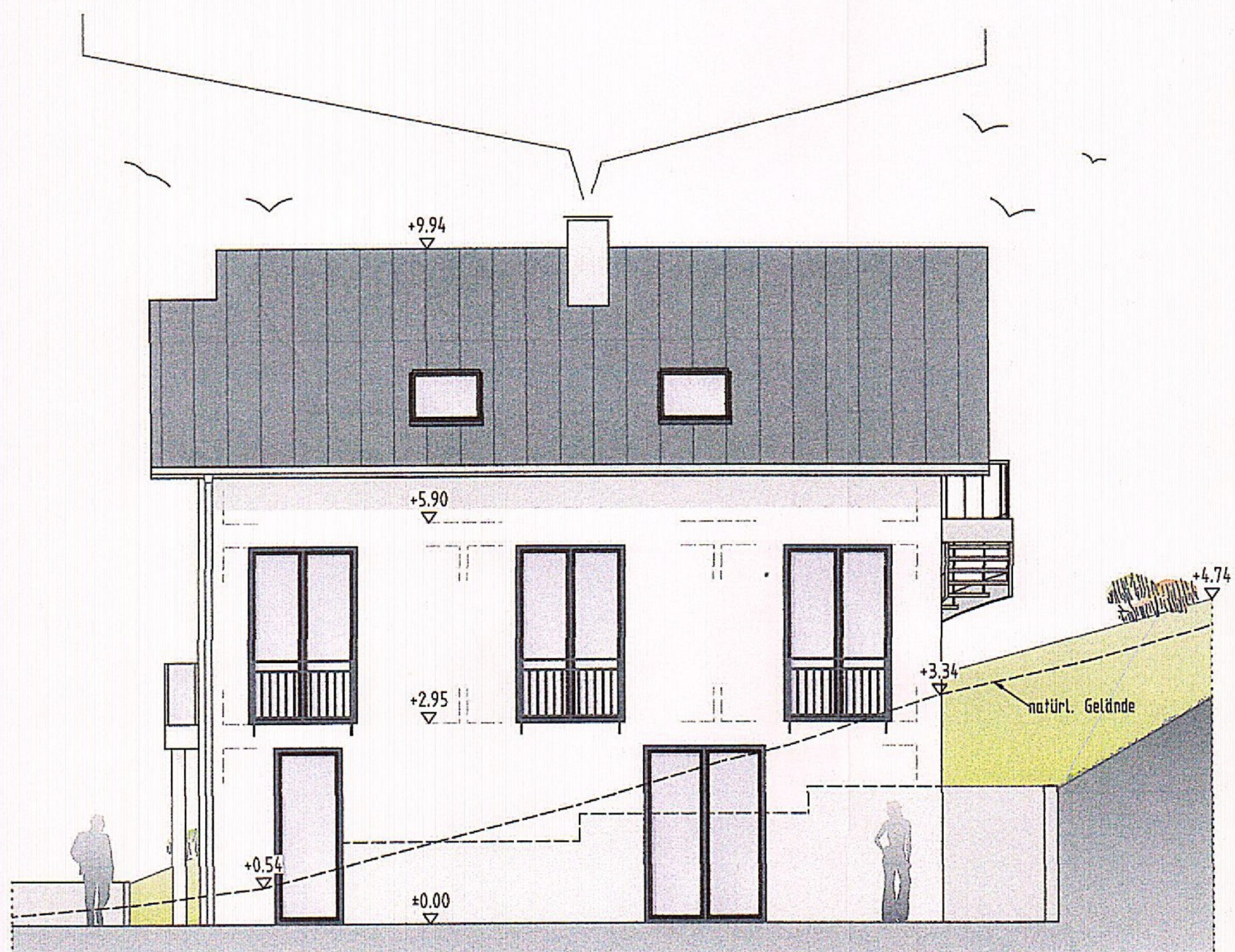
Ansicht West
