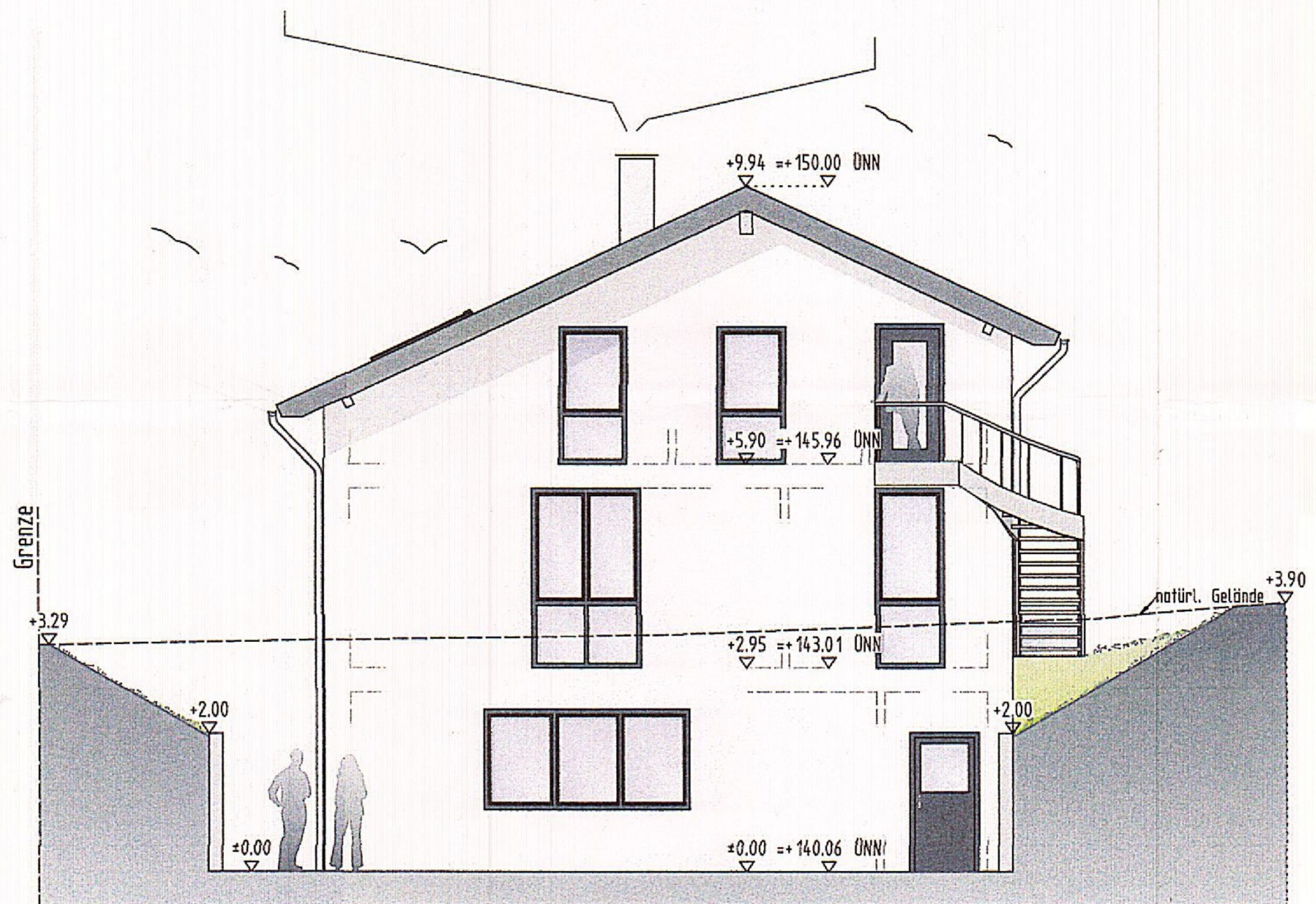
Ansicht Süd
