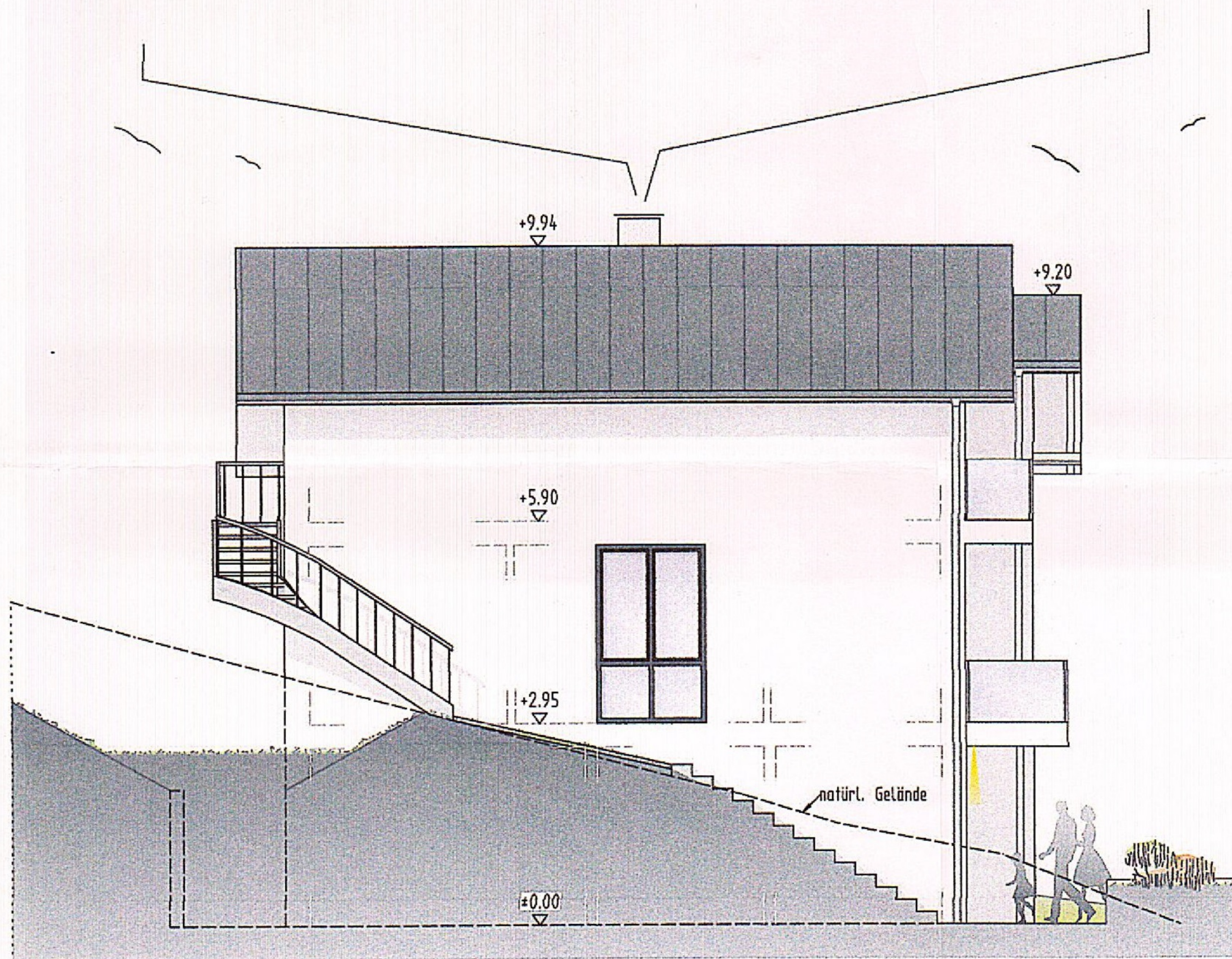
Ansicht Ost
