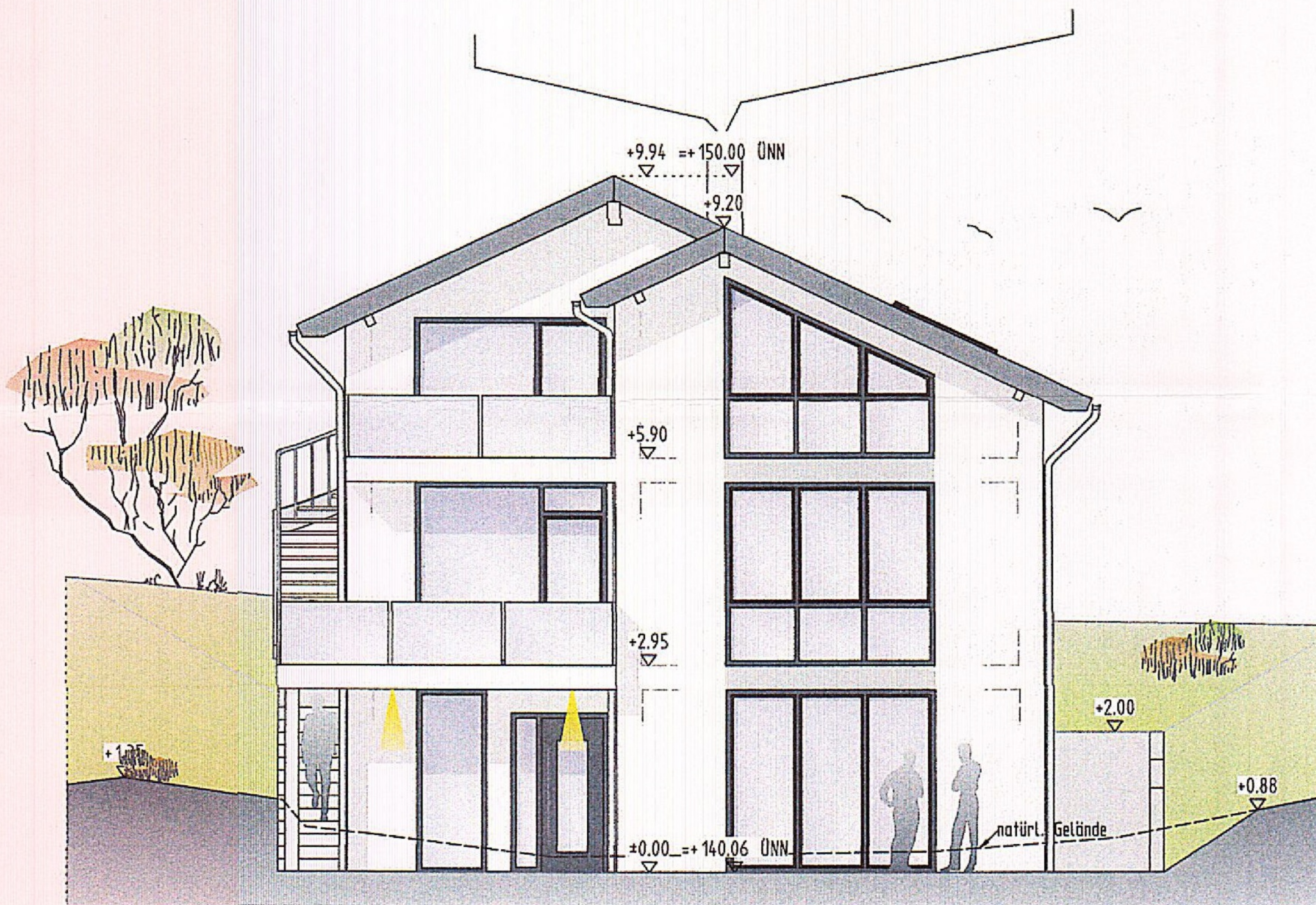
Ansicht Nord
