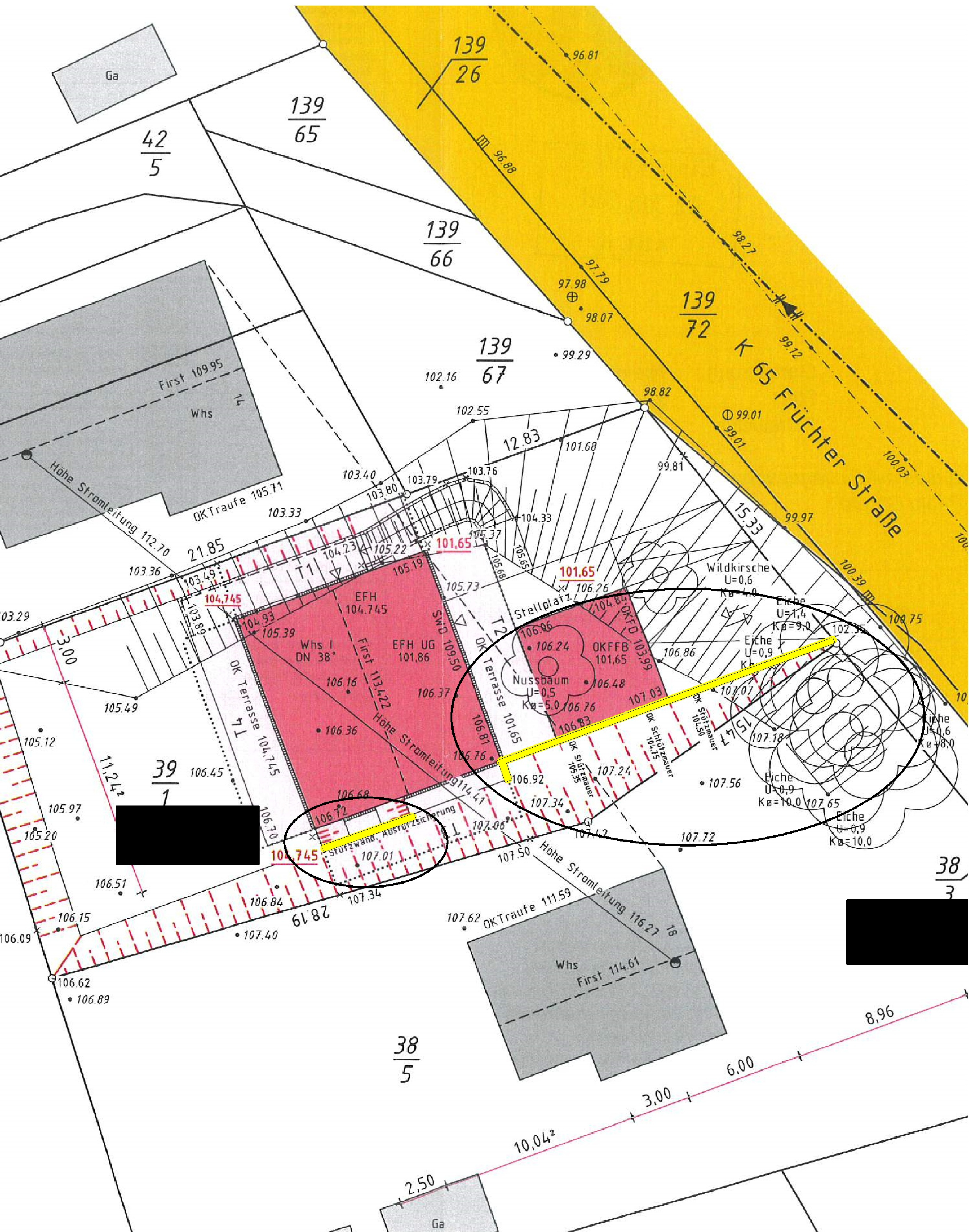
Lageplan - Stützmauer_alt (Genehmigungsplan)
