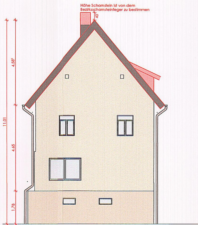
Ansicht Süd Rekonstruktion gem. Gutachten - Pfettendach mit Schleppgaube über Treppenraum
