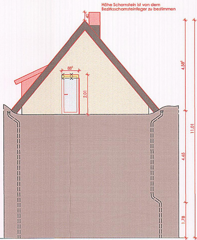
Ansicht Nord Rekonstruktion gem. Gutachten - Pfettendach mit Schleppgaube über Treppenraum
