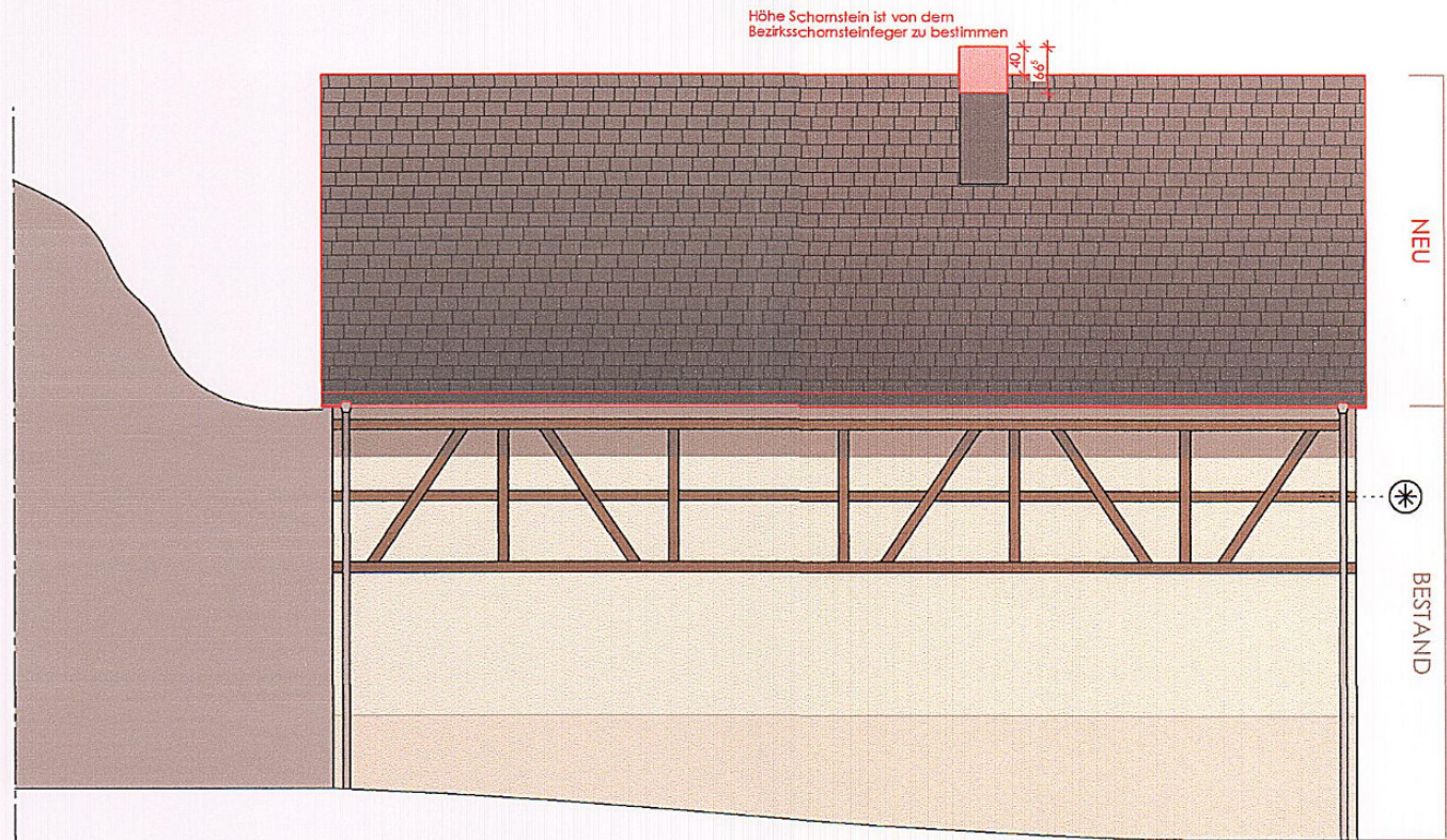
Ansicht West Rekonstruktion gem. Gutachten - Pfettendach mit Schleppgaube über Treppenraum
