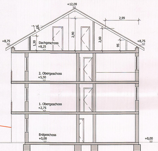
Querschnitt M 1:100
