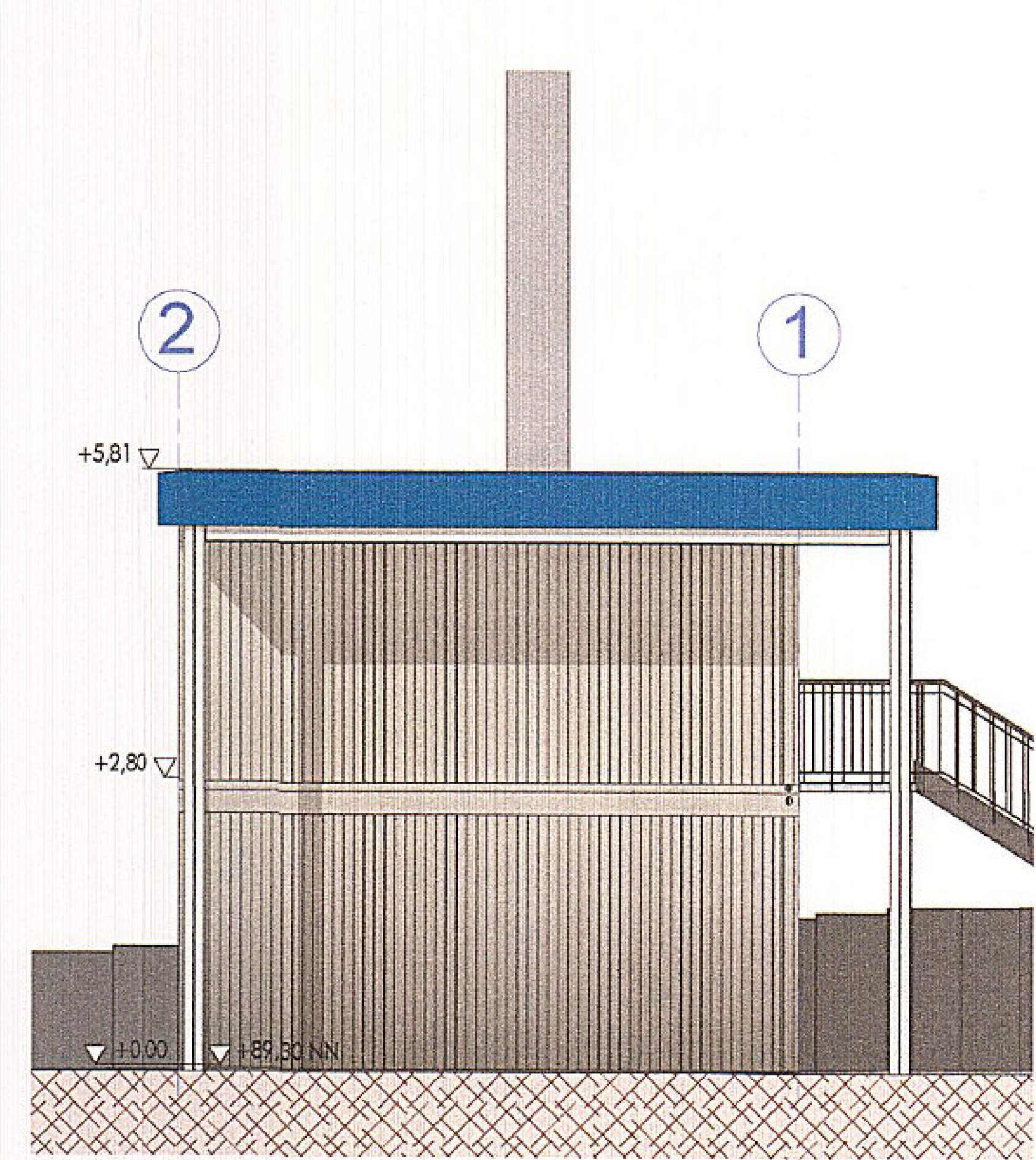
SÜD, M 1:100
