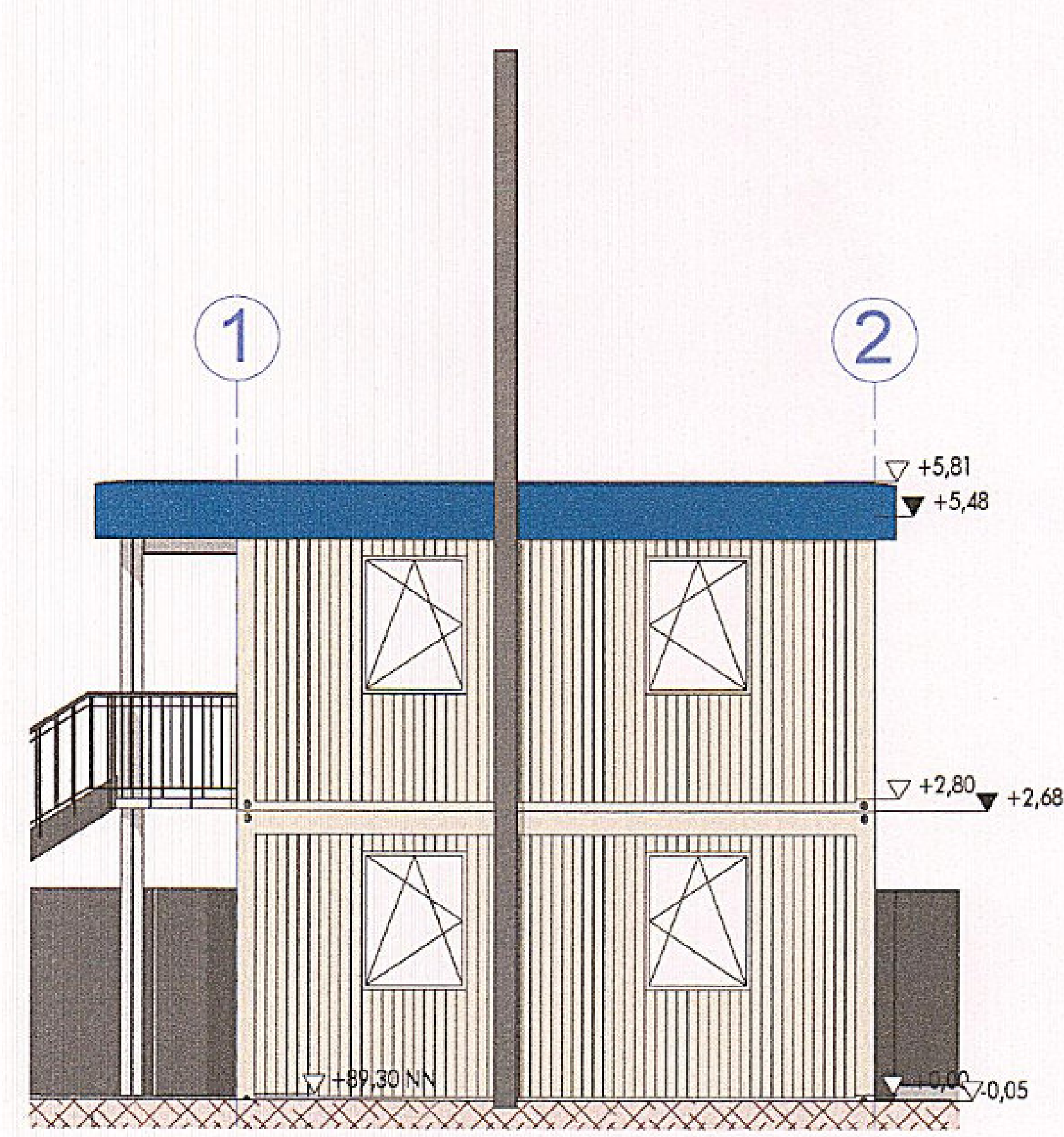
NORD, M 1:100
