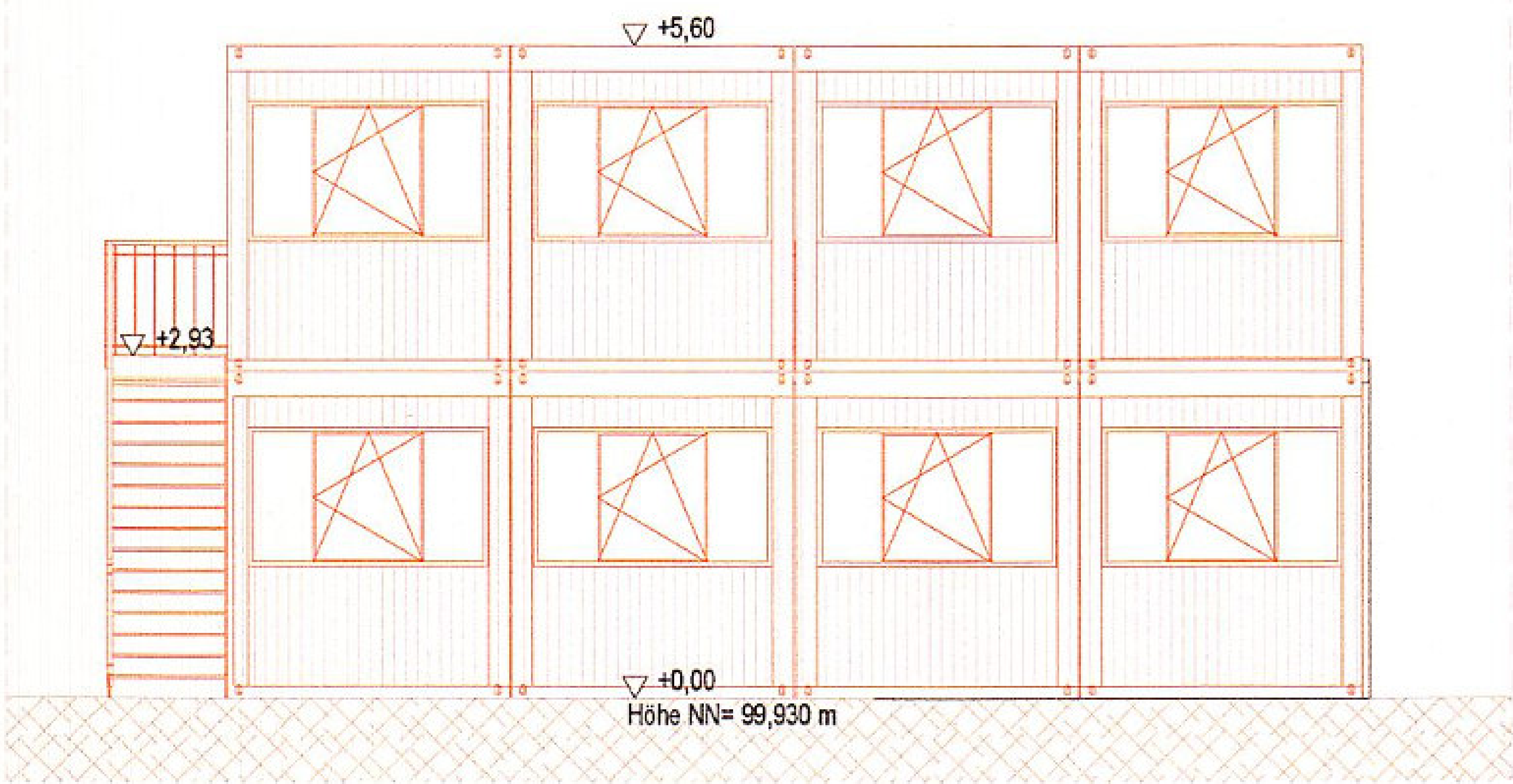
BÜROCONTAINER, ANSICHT NORD-WEST, M. 1:100
