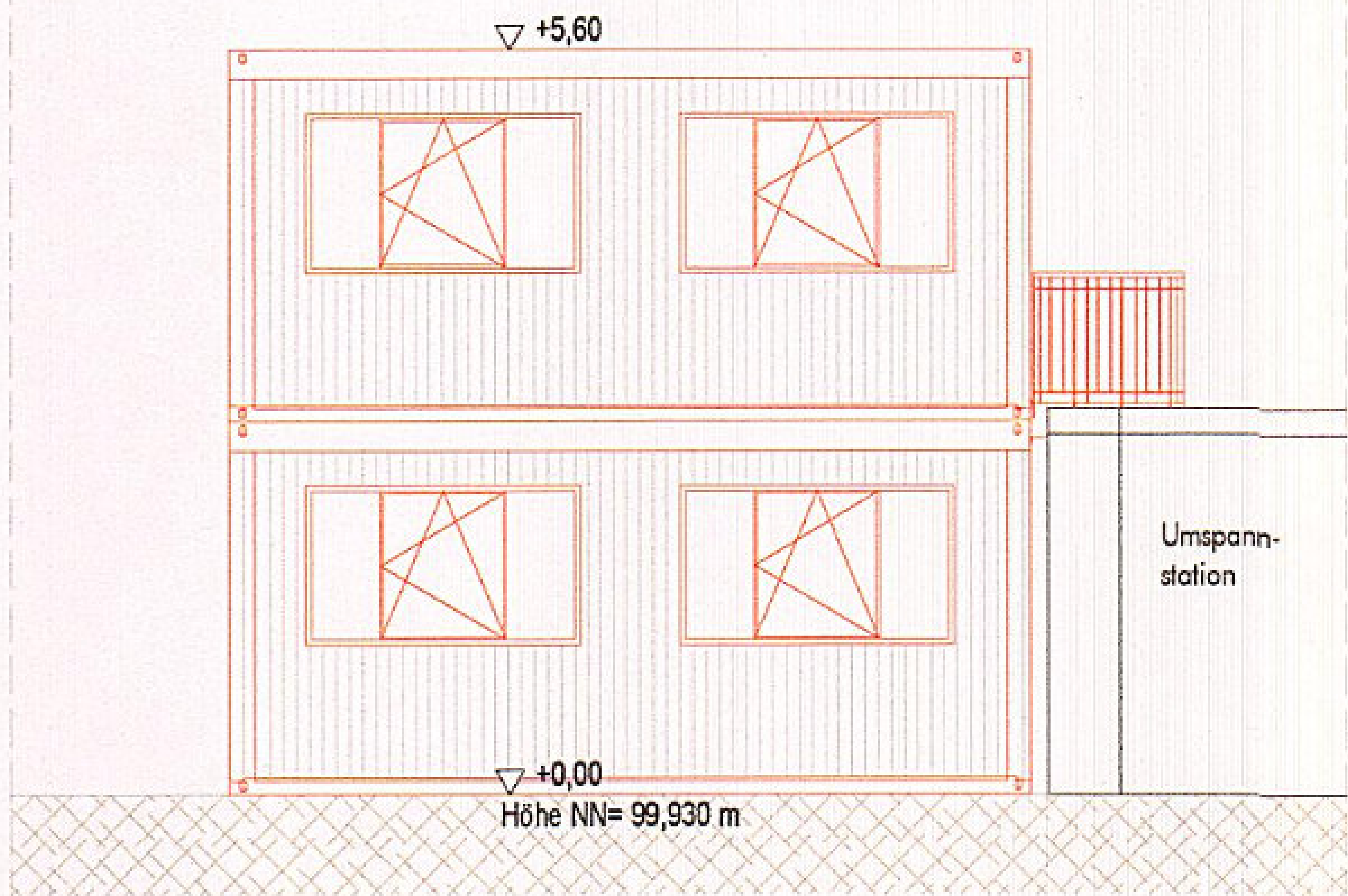
BÜROCONTAINER, ANSICHT SÜD-WEST, M. 1:100
