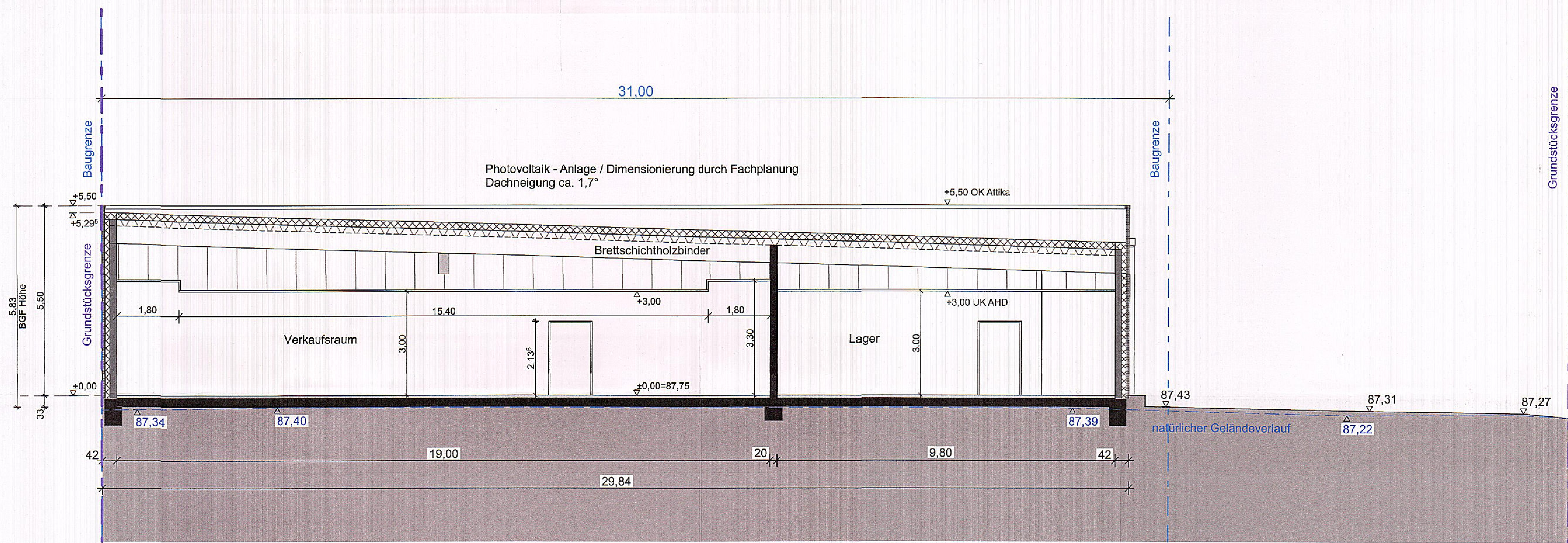
Schnitt A-A
