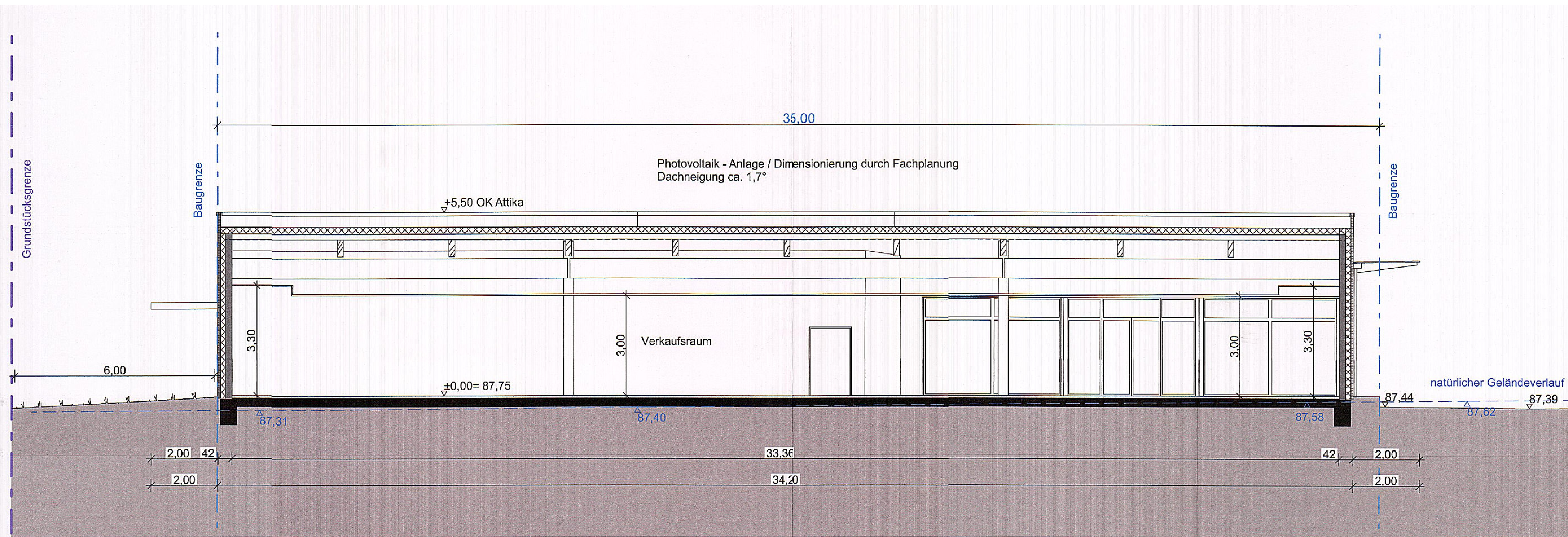
Schnitt B-B
