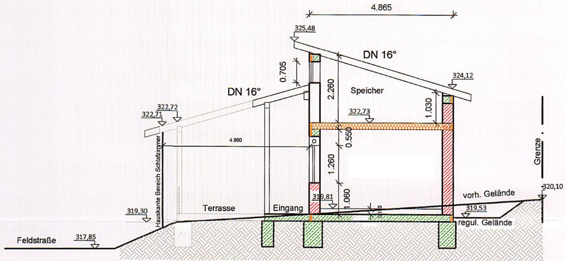
Querschnitt durch Eingang
