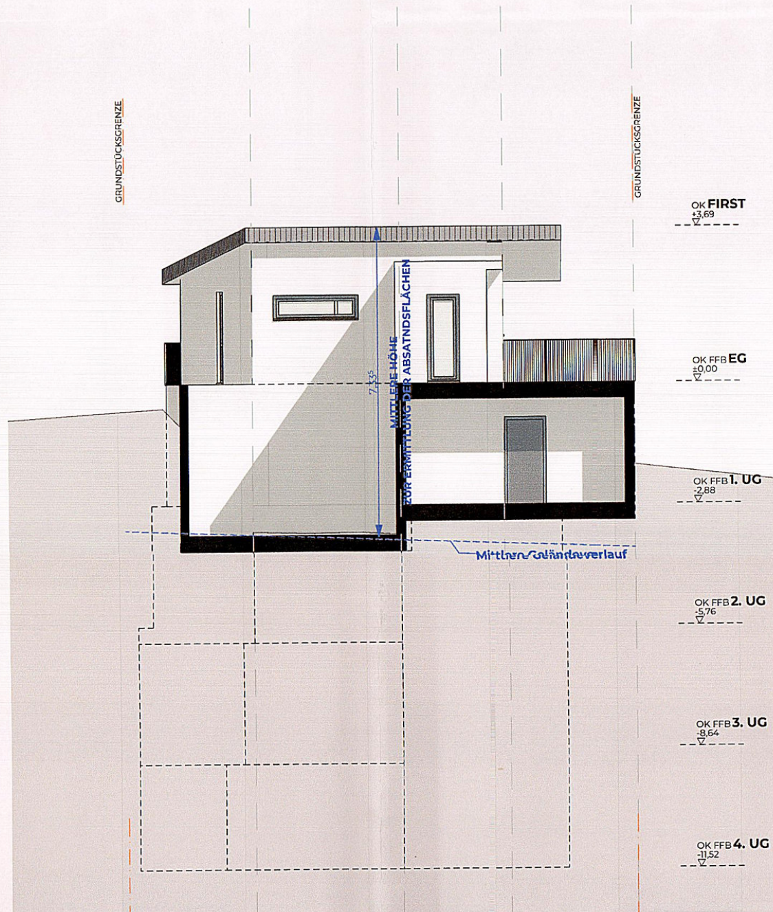
ANSICHT OST
