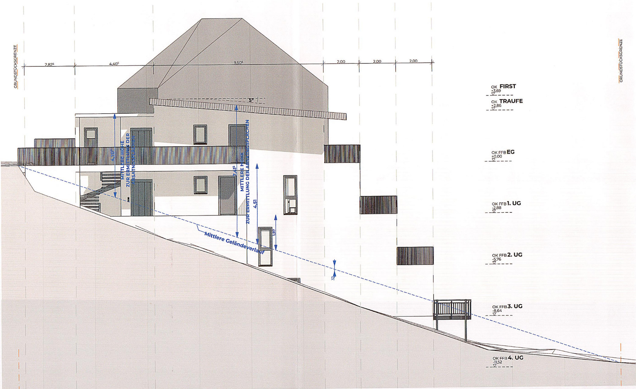
ANSICHT NORD
