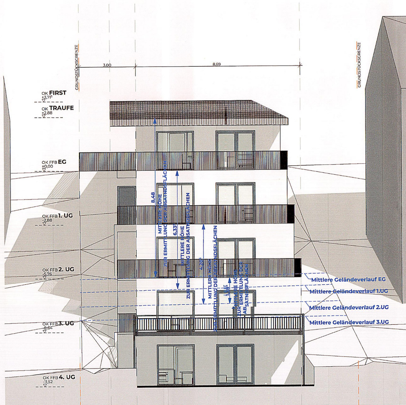
ANSICHT WEST
