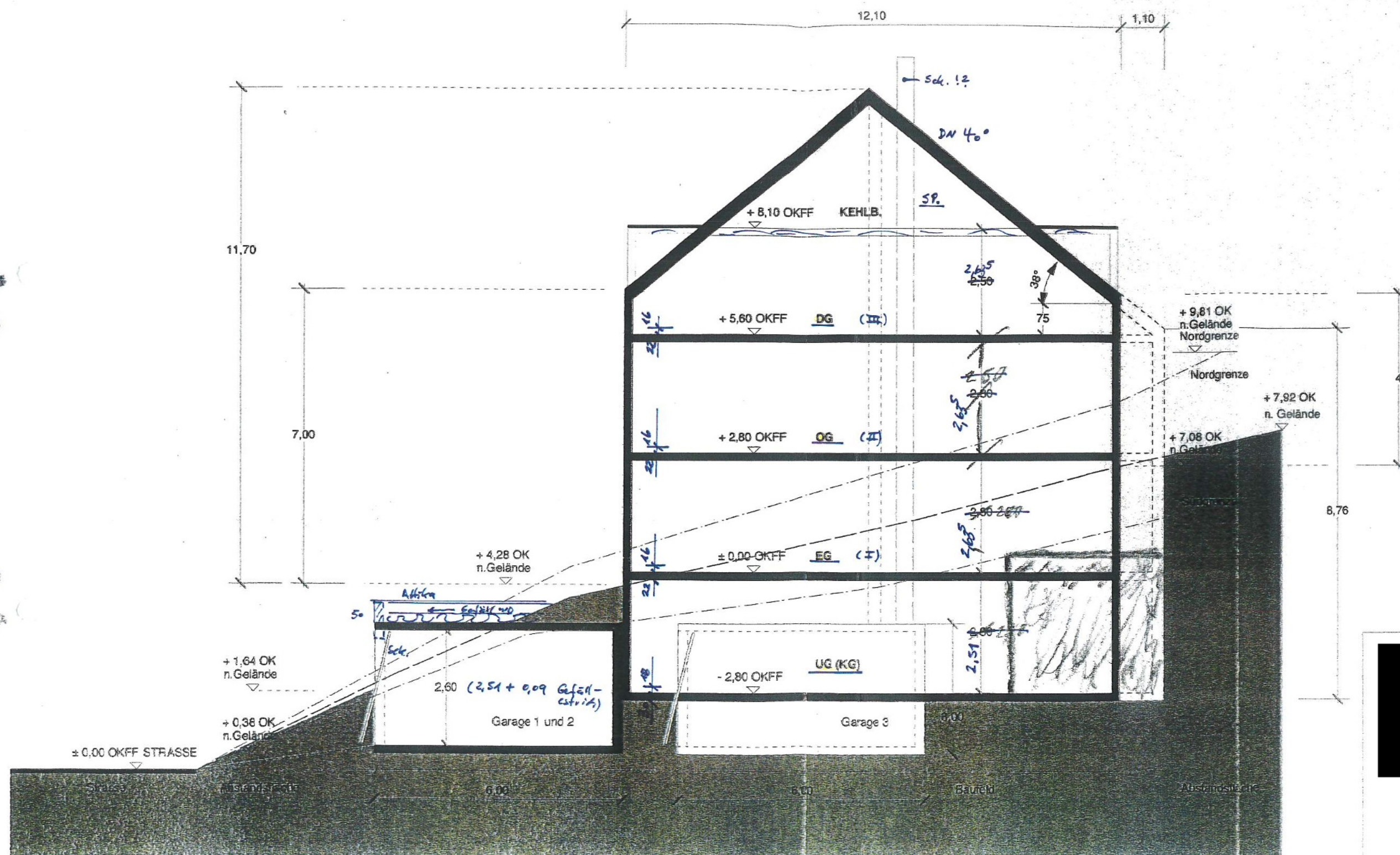
SCHNITT A-A
