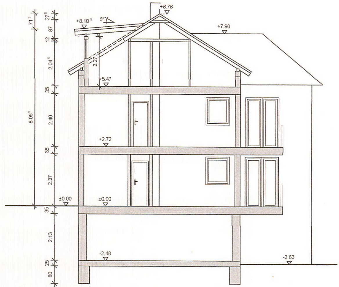
SCHNITT A-A
