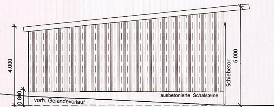
Ansicht von Süd Osten unverändert
