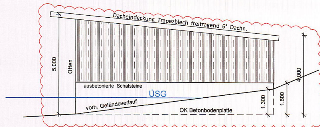
Ansicht von Nord Westen
