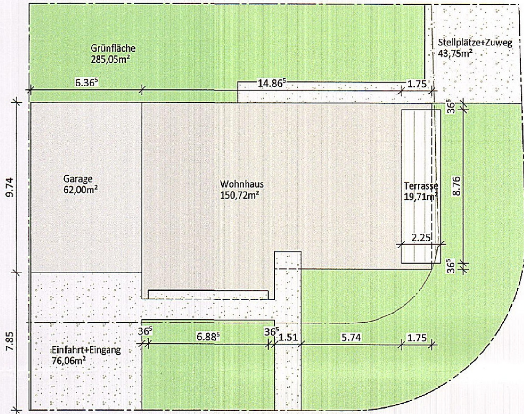
Freiflächenplan M XXXXXXXXXX
