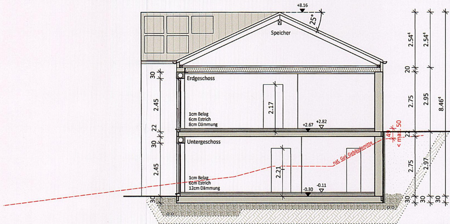
Schnitt A-A
