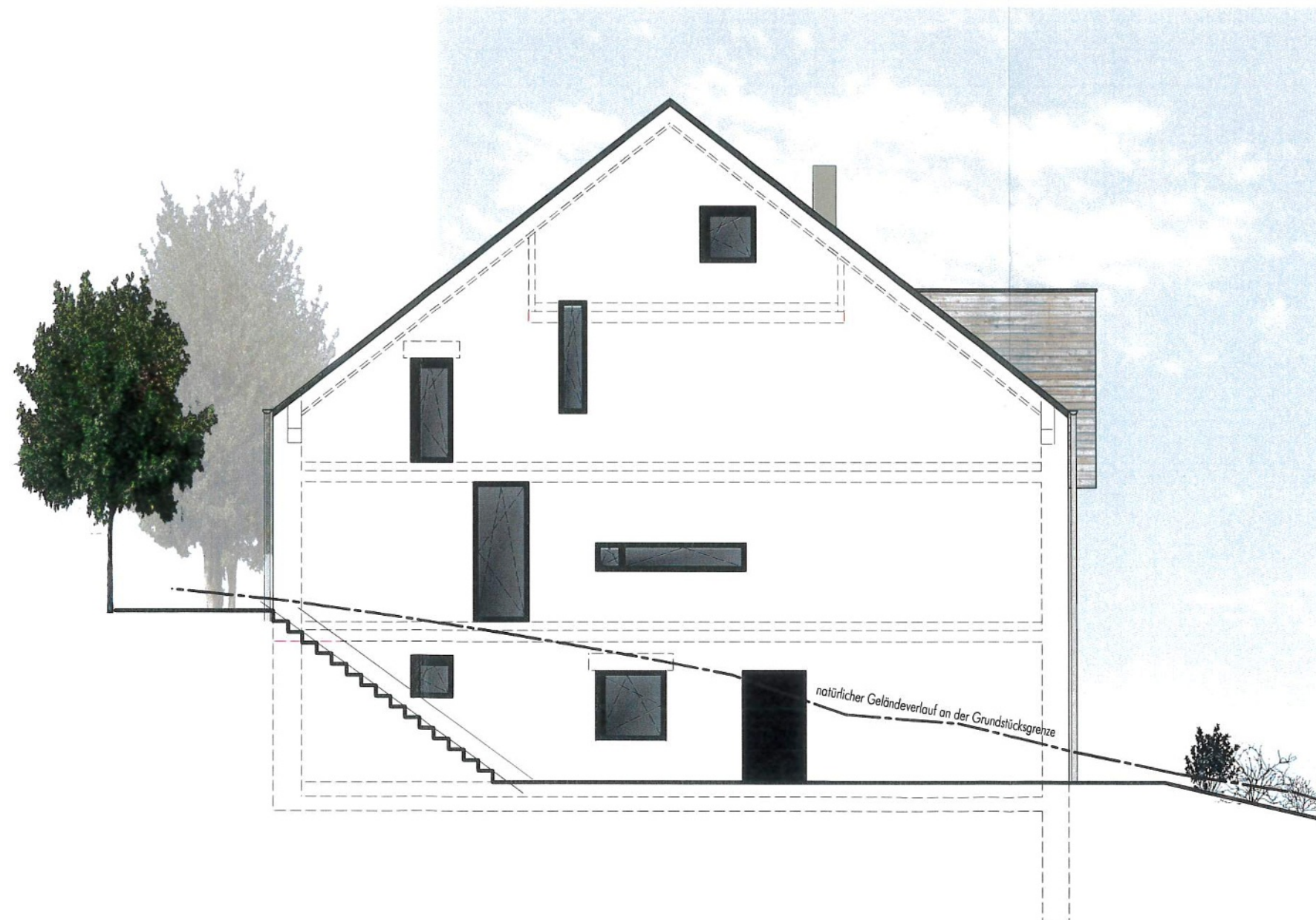
Ansicht Nord-Ost
