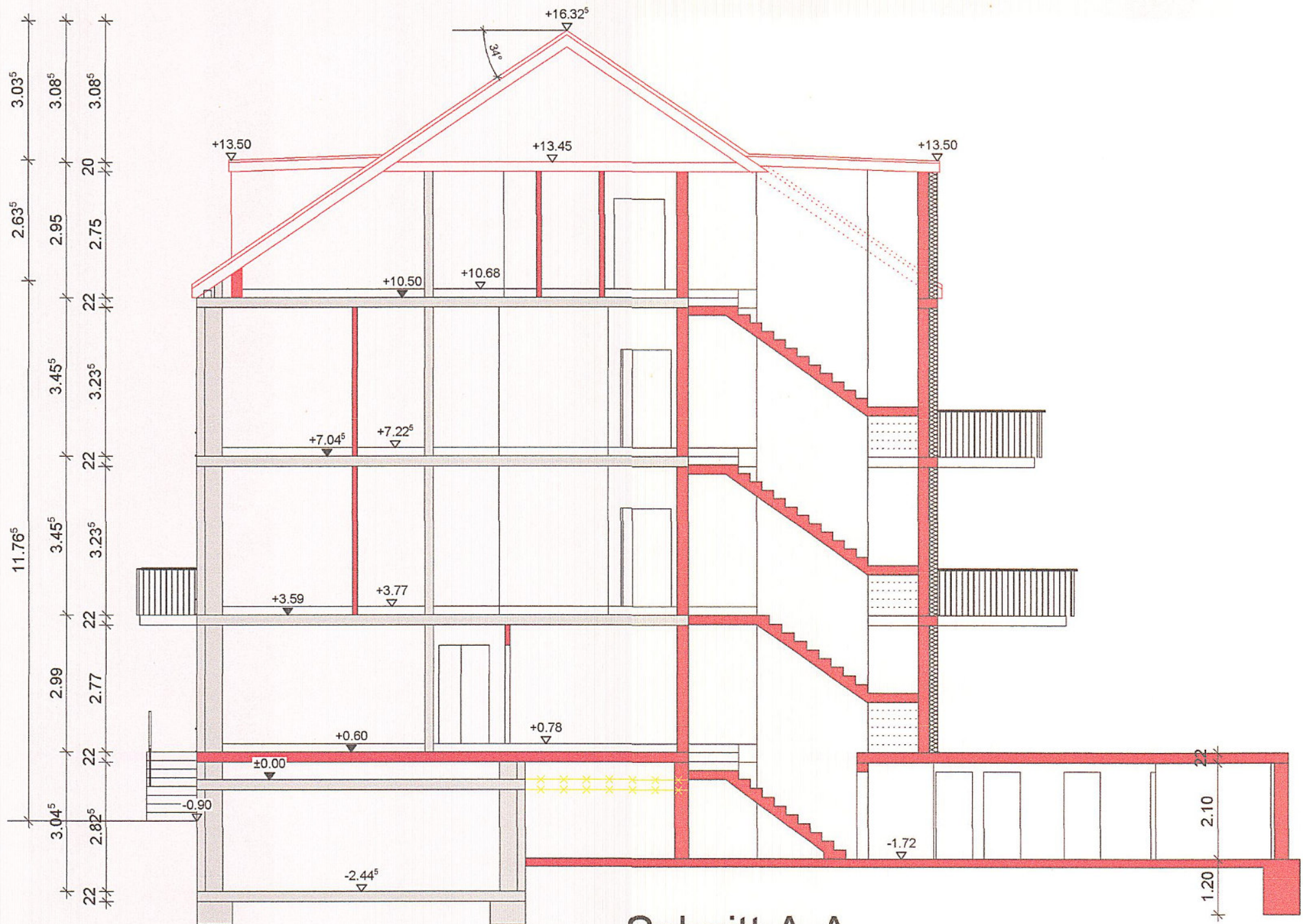
Schnitt A-A
