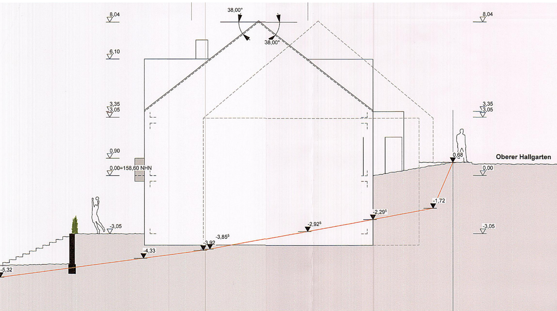
Ansicht Süd-Ost
