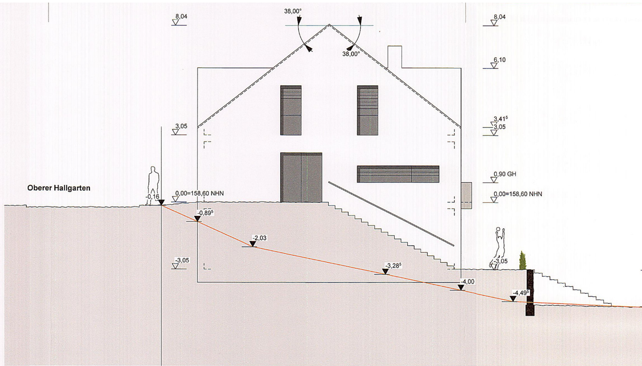
Ansicht Nord-West
