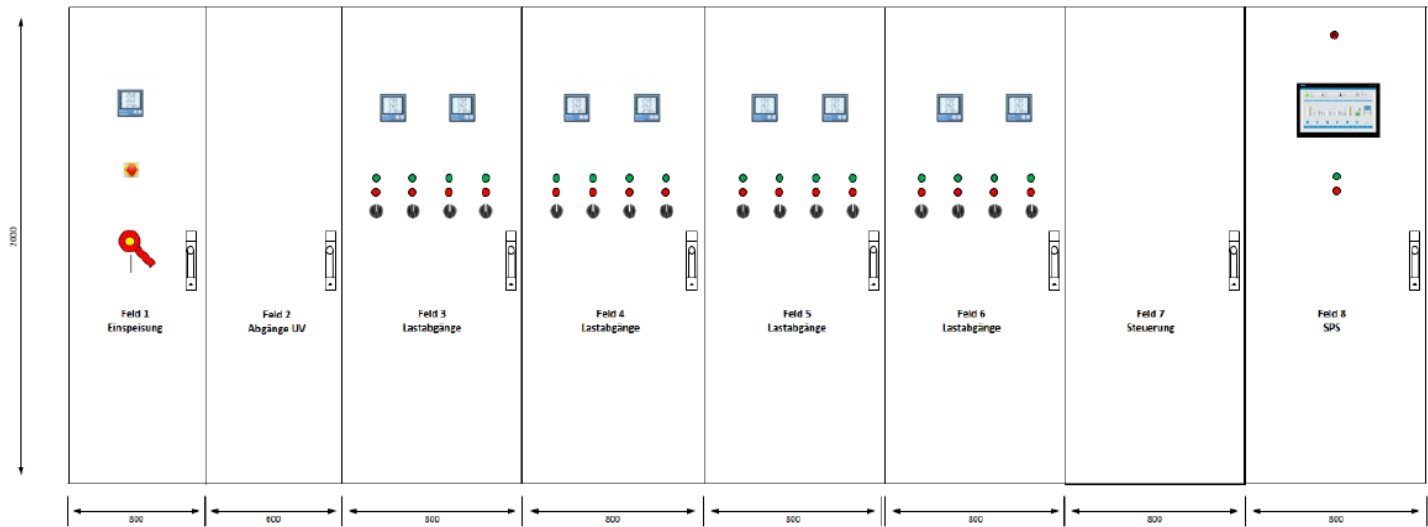
NSHV KA Langenau
