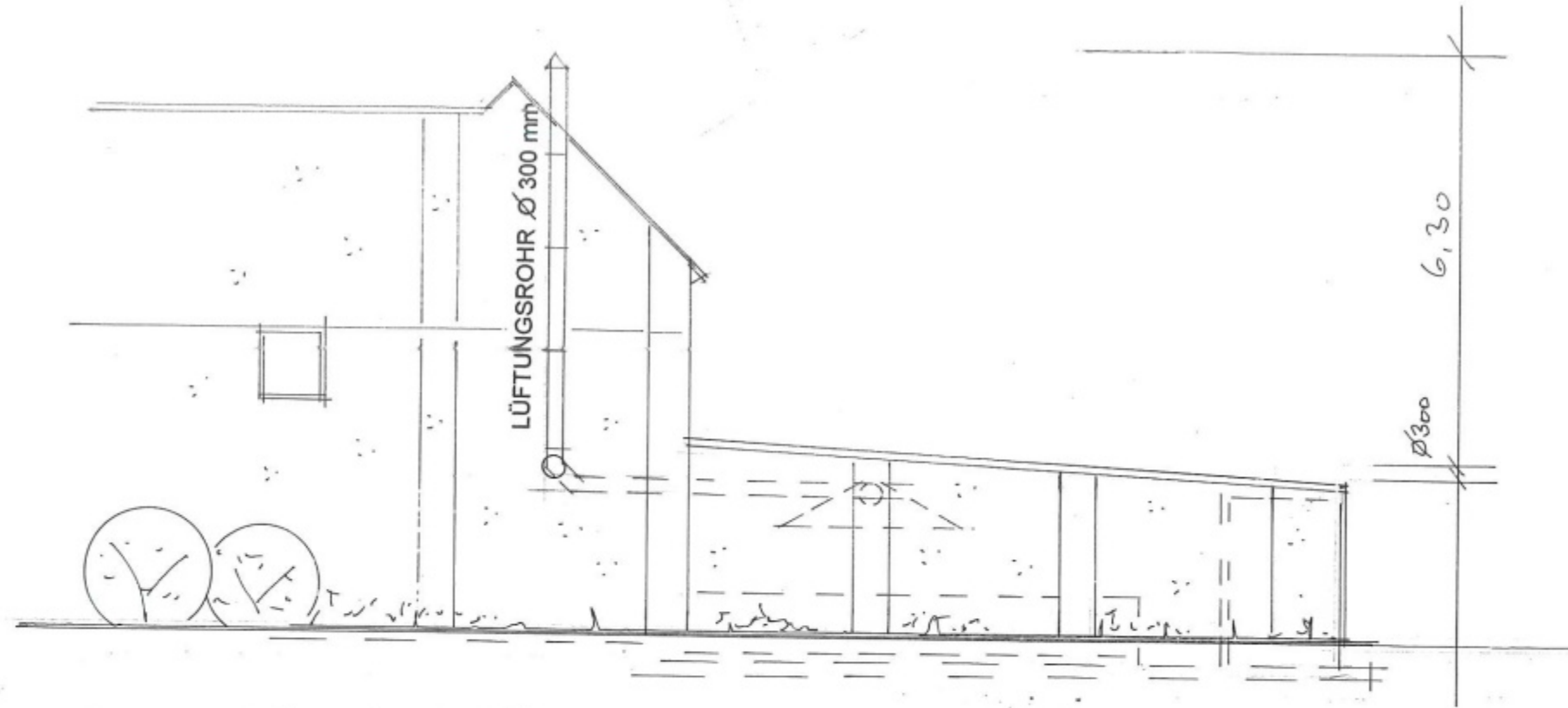
NORD-ANSICHT
