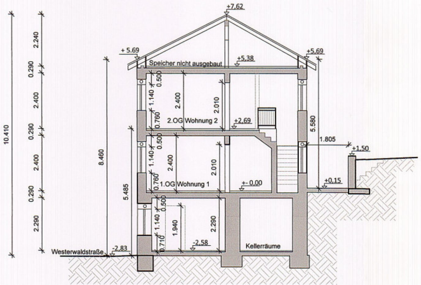
Querschnitt A - A
