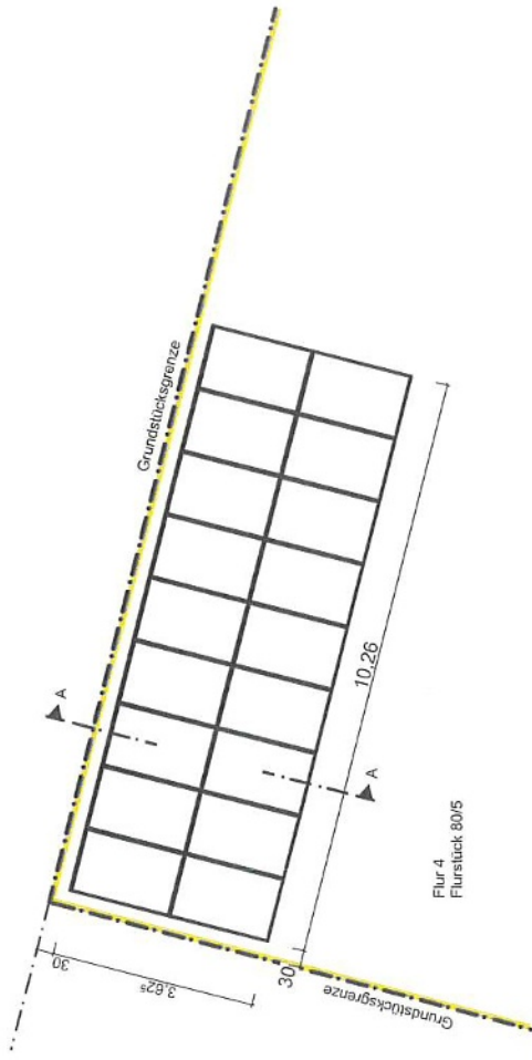
Grundriss_PV-Anlage M 1:100
