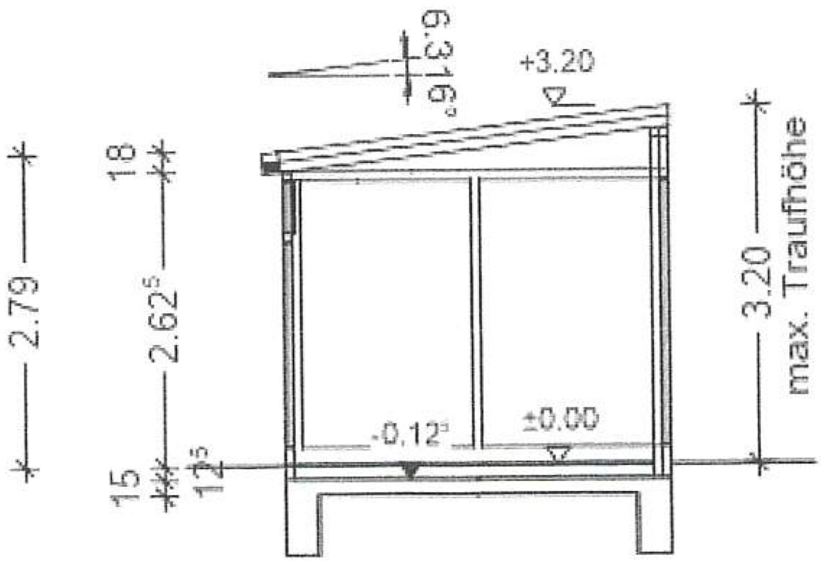
Schnitt B-B
