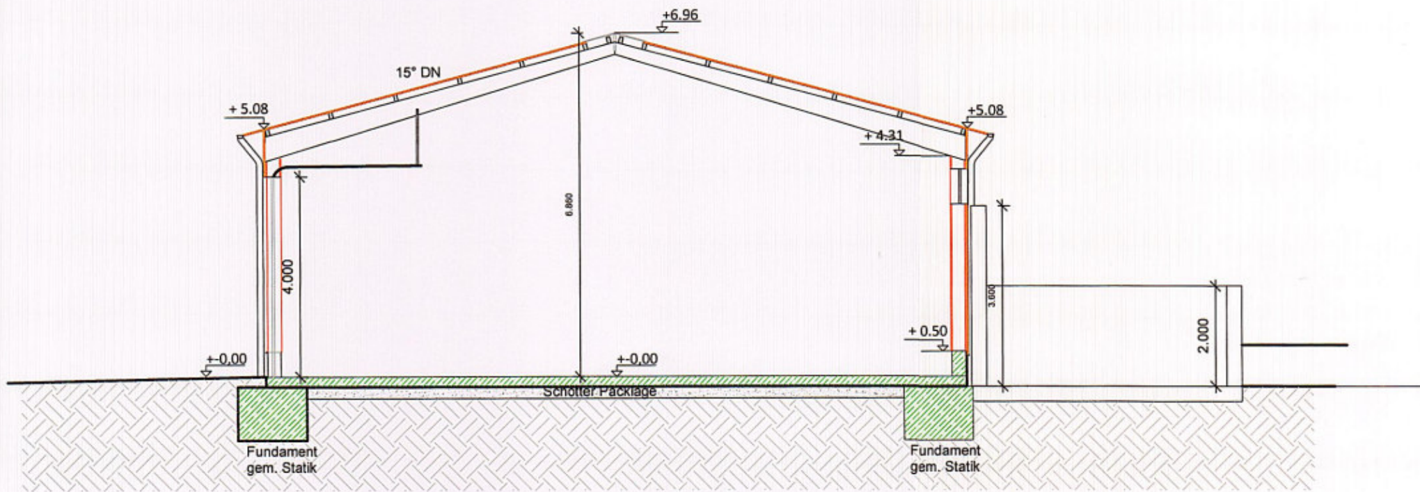
Querschnitt
