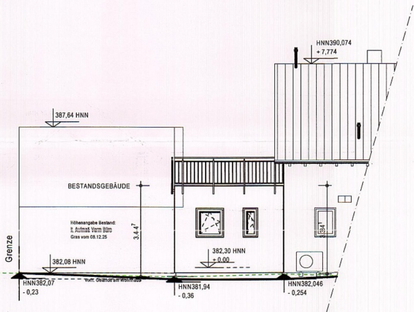
Ansicht Nordosten M 1:100
