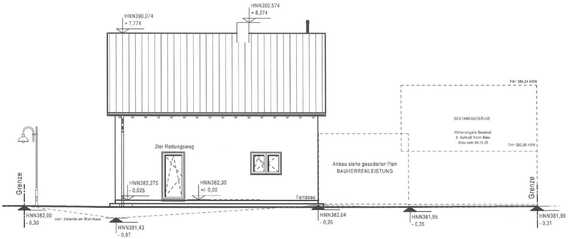
Ansicht von Nordwesten M 1:100
