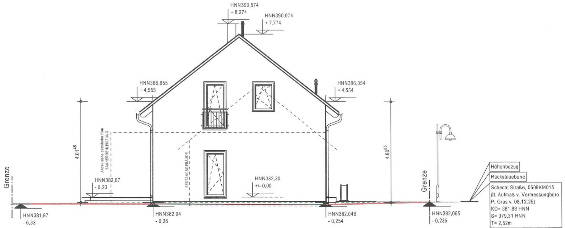
Ansicht von Südwesten M 1:100
