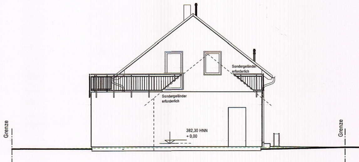
Ansicht Südosten M 1:100
