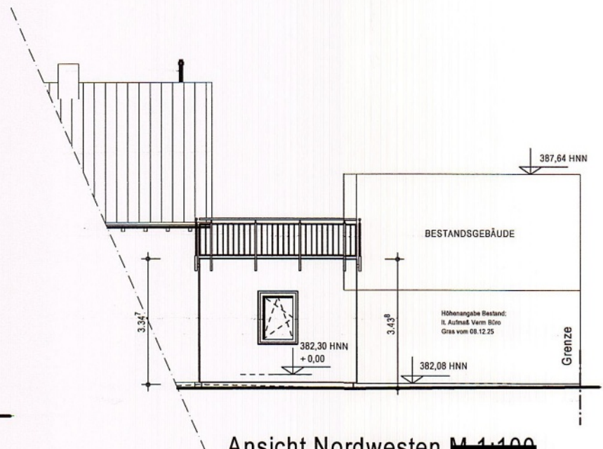
Ansicht Nordwesten M 1:100
