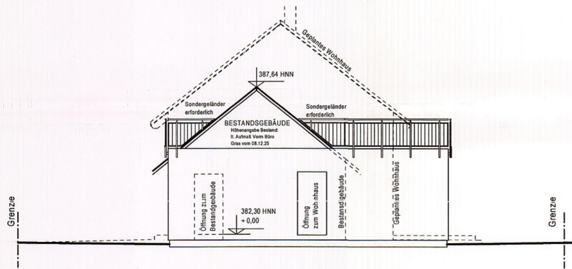
Ansicht Südwesten M 1:100
